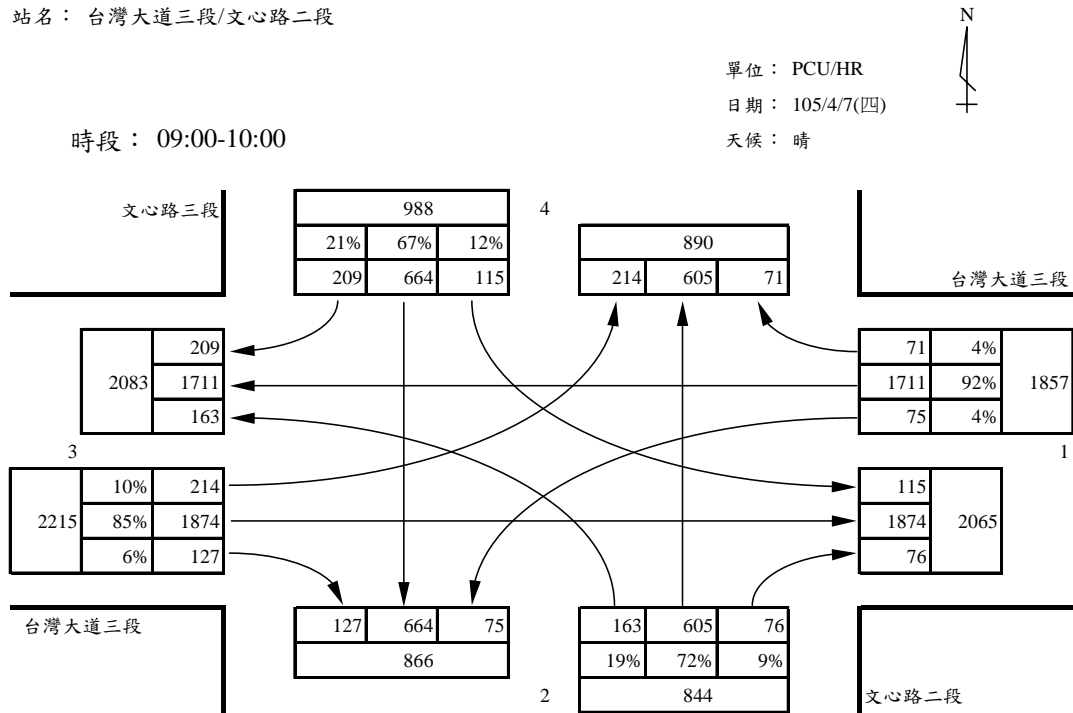
圖 2.3-6 文心路三段/臺灣大道三段路口轉向交通量圖
