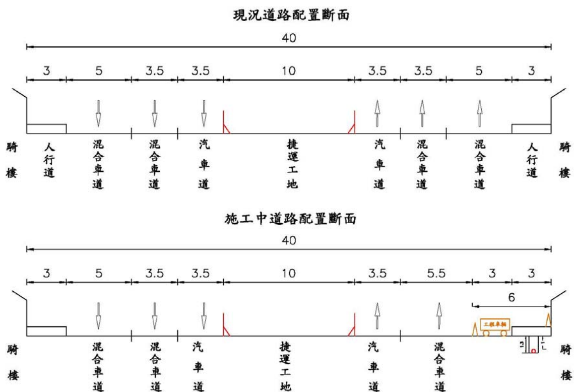
圖 4.2-1 施工中道路配置斷面圖
