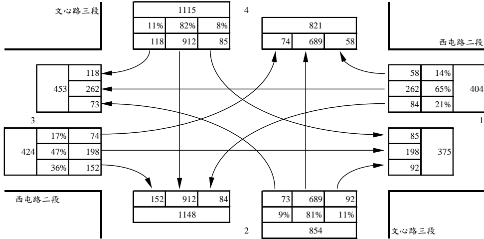
圖 2.3-2 文心路三段/西屯路二段路口轉向交通量圖
