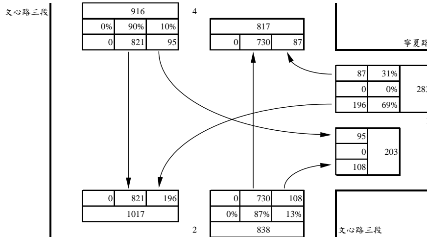
圖 2.3-4 文心路三段/寧夏路路口轉向交通量圖
