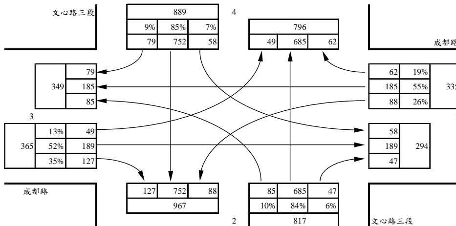
圖 2.3-5 文心路三段/成都路路口轉向交通量圖
