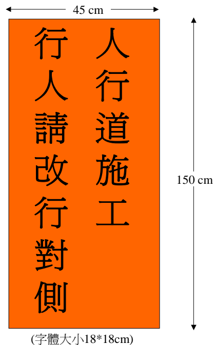
圖 4.4-1 行人改道標誌牌面尺寸
