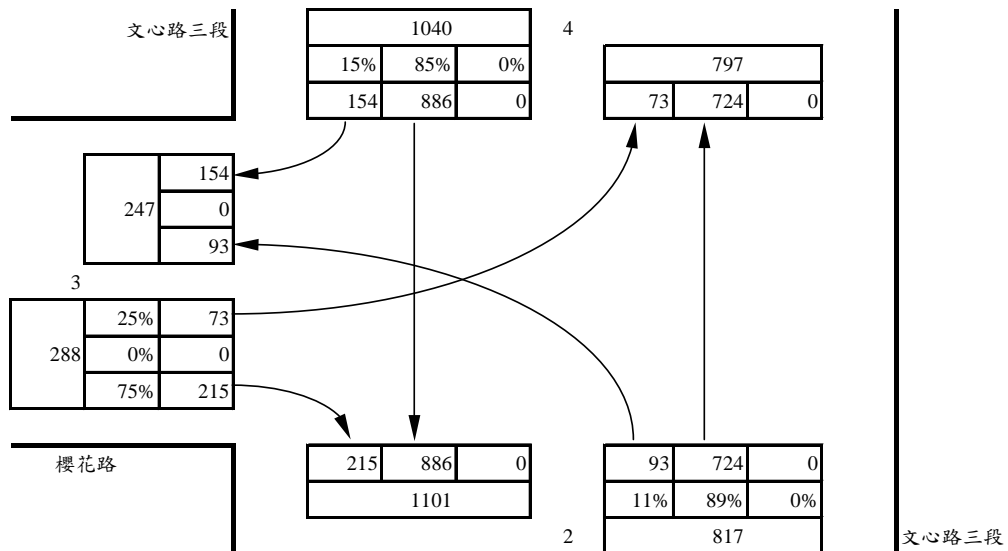
圖 2.3-3 文心路三段/櫻花路路口轉向交通量圖
