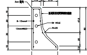
紐澤西護欄
