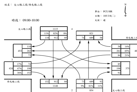
圖 2.3-1 路口服務水準評估軟體示意圖
