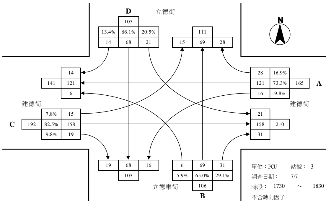
立德東街與建德街路口平日昏峰轉向交通量示意圖
