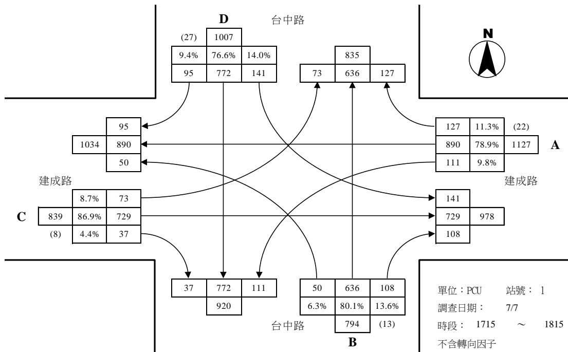
台中路與建成路路口平日昏峰轉向交通量示意圖
