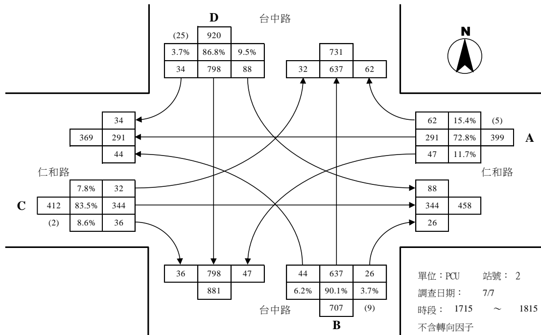
台中路與仁和路路口平日昏峰轉向交通量示意圖
