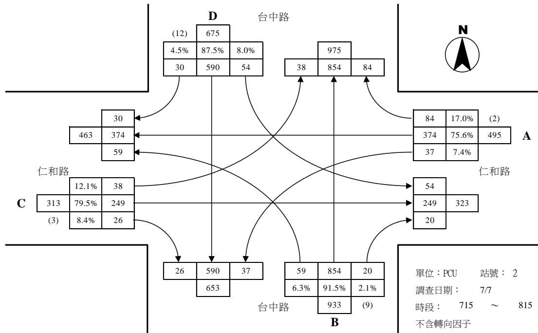
台中路與仁和路路口平日晨峰轉向交通量示意圖
