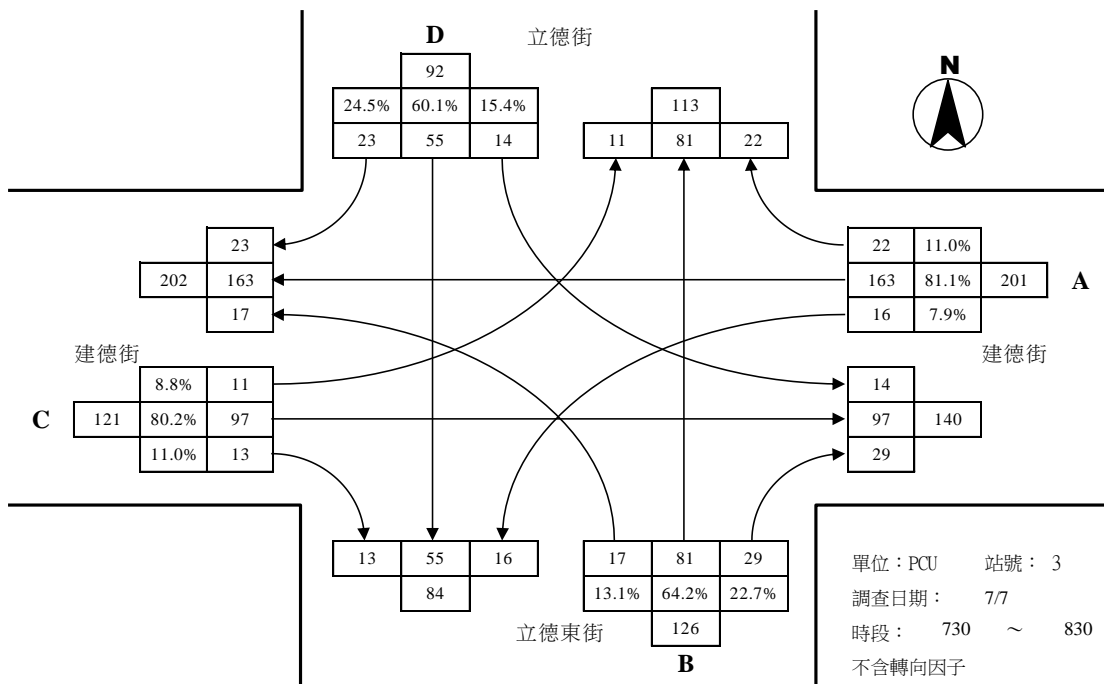
立德東街與建德街路口平日晨峰轉向交通量示意圖
