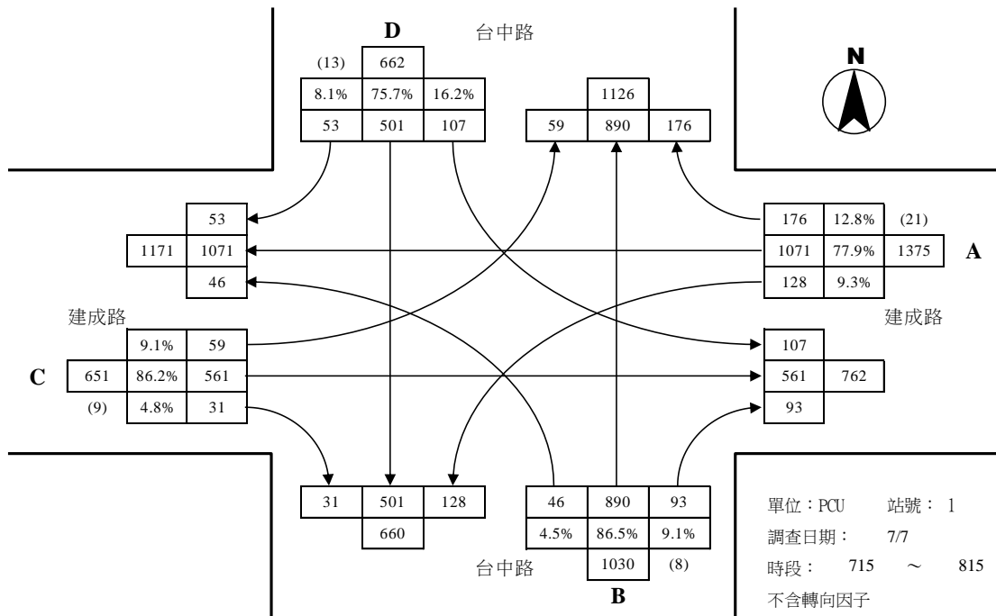
台中路與建成路路口平日晨峰轉向交通量示意圖
