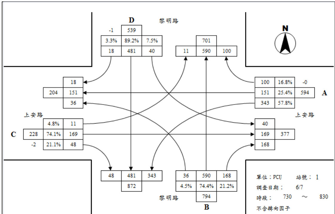
黎明路與上安路路口平日晨峰轉向交通量示意圖
