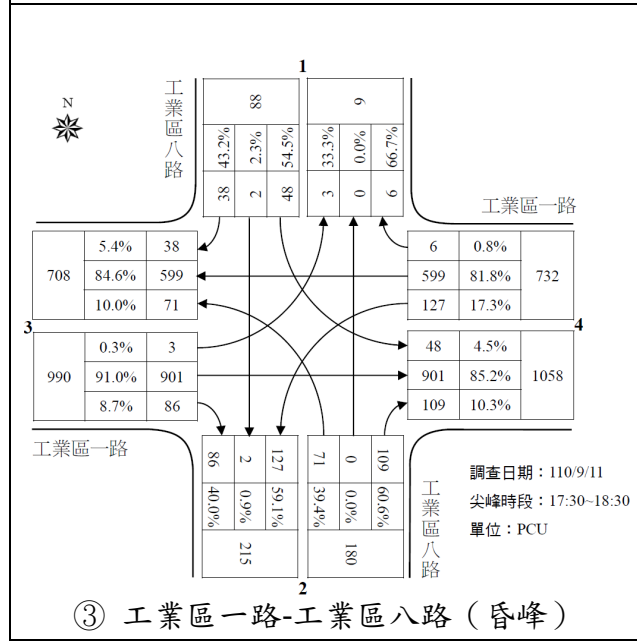
基地周邊主要路口尖峰時段交通量示意圖-假日 (續)
