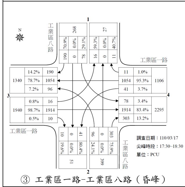
基地周邊主要路口尖峰時段交通量示意圖-平日 (續)
