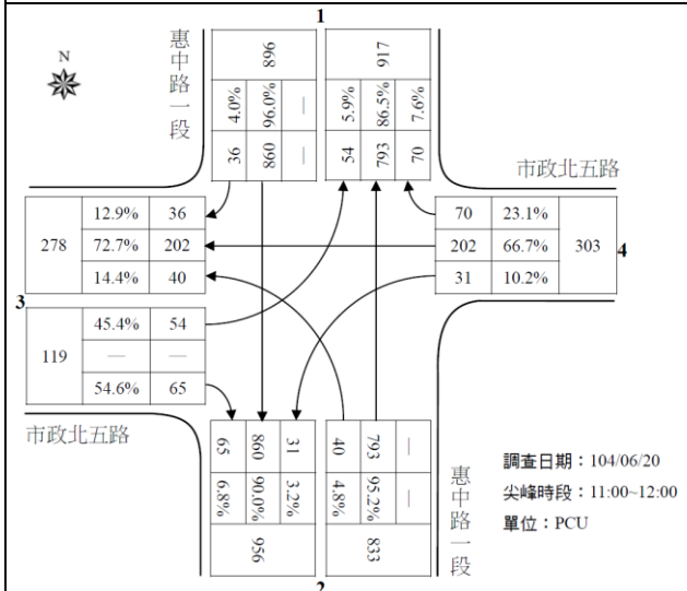
惠中路一段-市政北五路 (假日晨峰)
