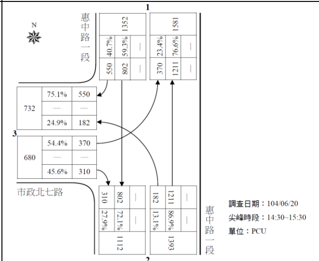
惠中路一段-市政北七路 (假日昏峰)
