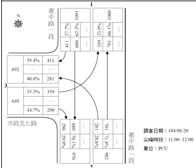
惠中路一段-市政北七路 (假日晨峰)
