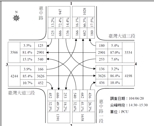
惠中路一段-臺灣大道三段 (假日昏峰)
