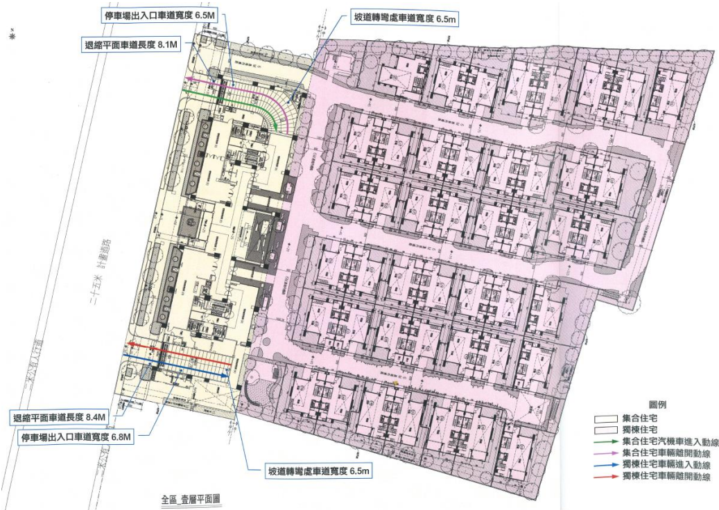
停車場出入 動線示意圖
