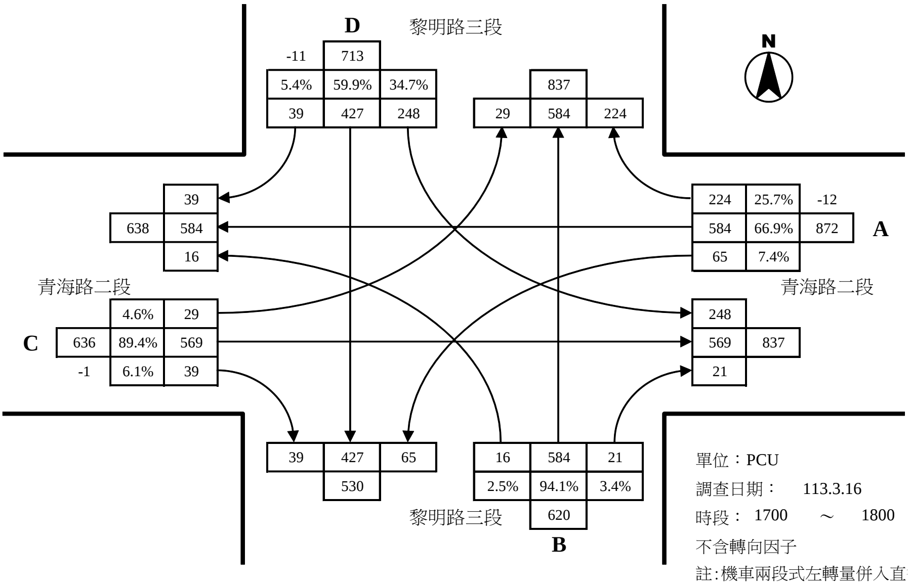
黎明路三段與青海路二段路口假日尖峰轉向交通量示意圖
