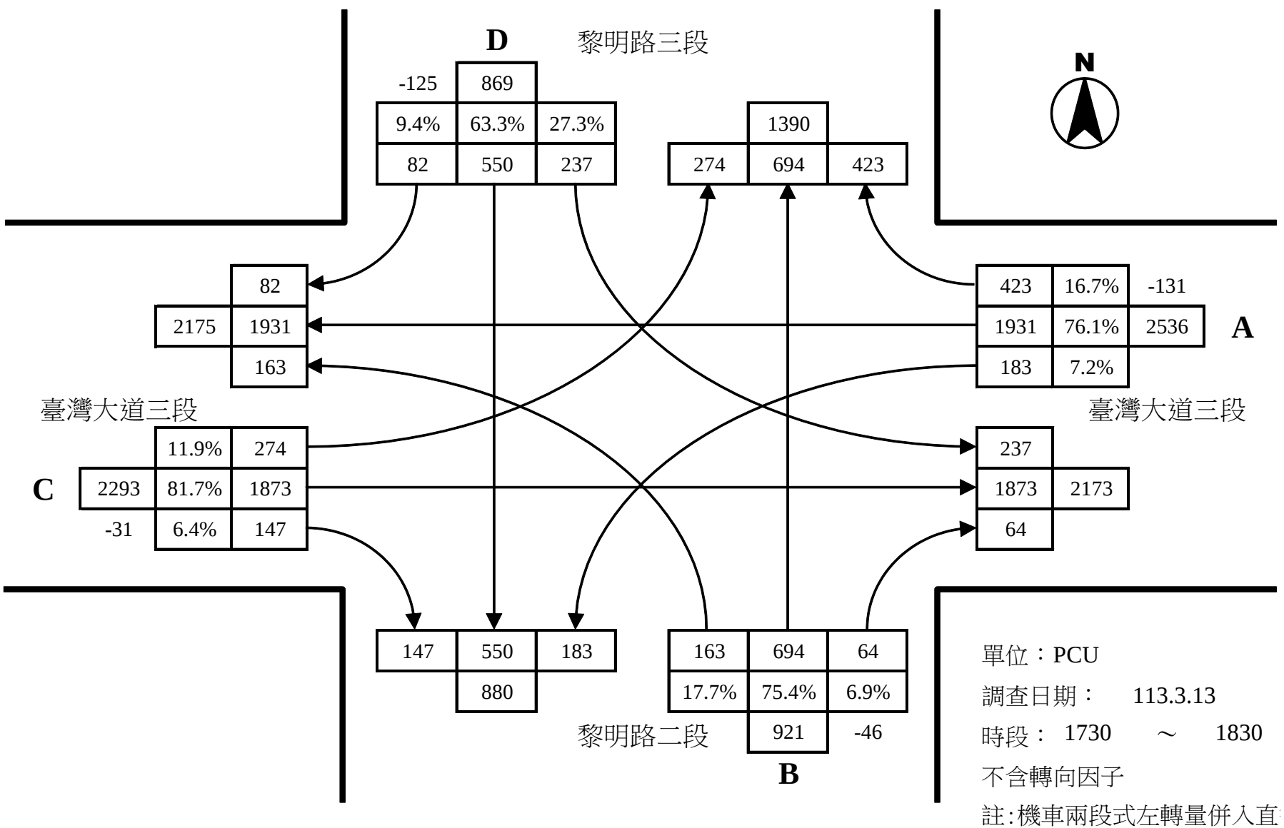
黎明路三段與臺灣大道三段路口平日昏峰轉向交通量示意圖
