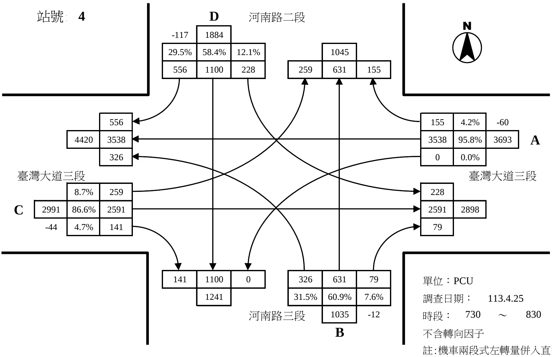
河南路二段與臺灣大道三段路口平日晨峰轉向交通量示意圖
