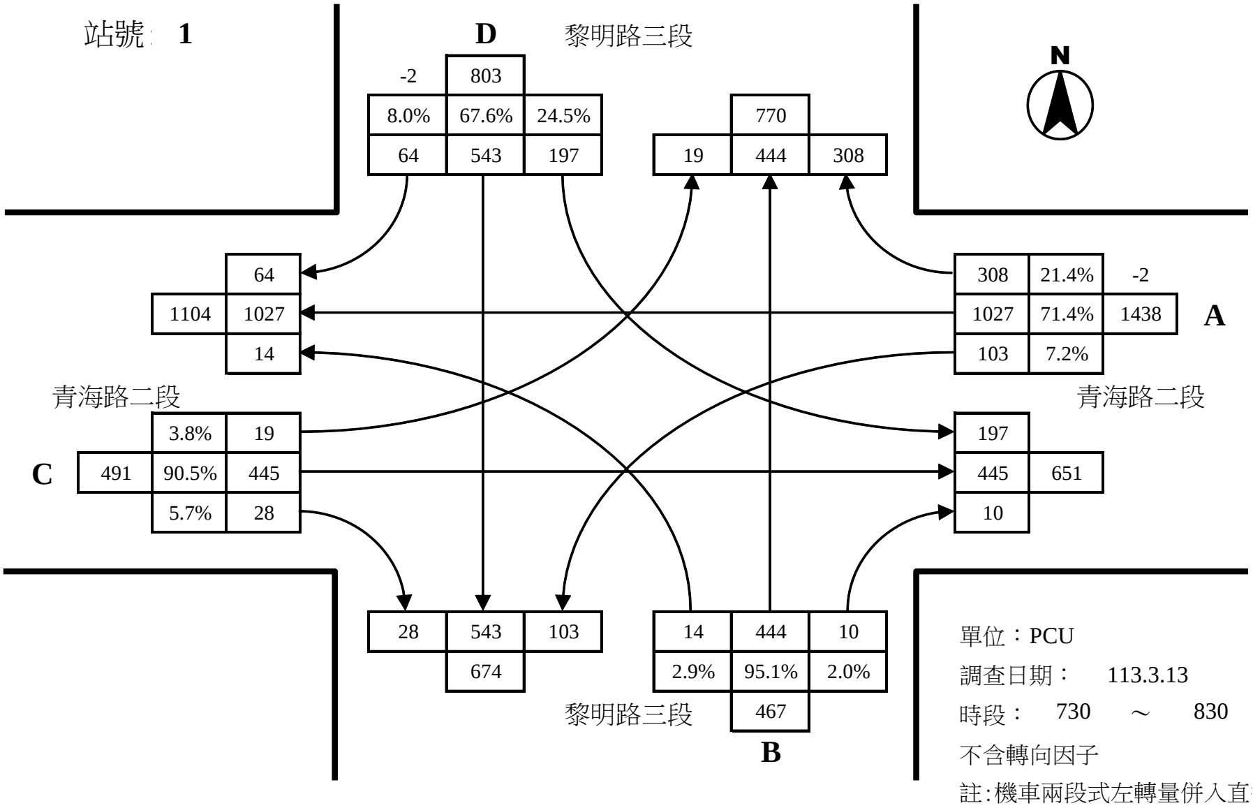
黎明路三段與青海路二段路口平日晨峰轉向交通量示意圖
