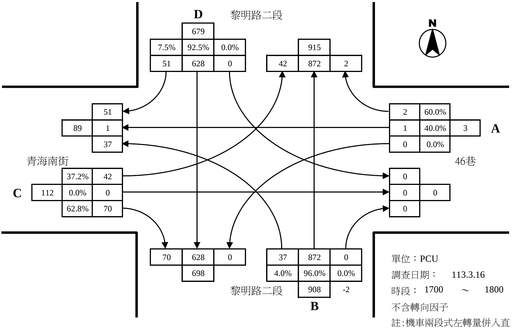
黎明路二段與青海南街路口假日尖峰轉向交通量示意圖
