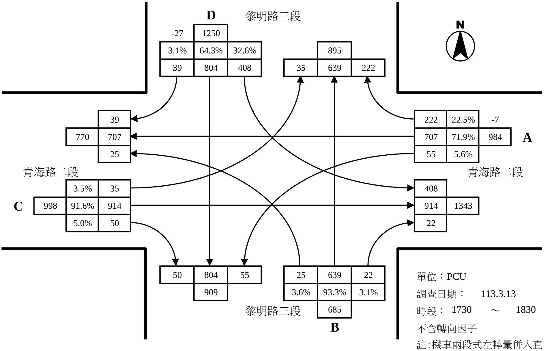
黎明路三段與青海路二段路口平日昏峰轉向交通量示意圖
