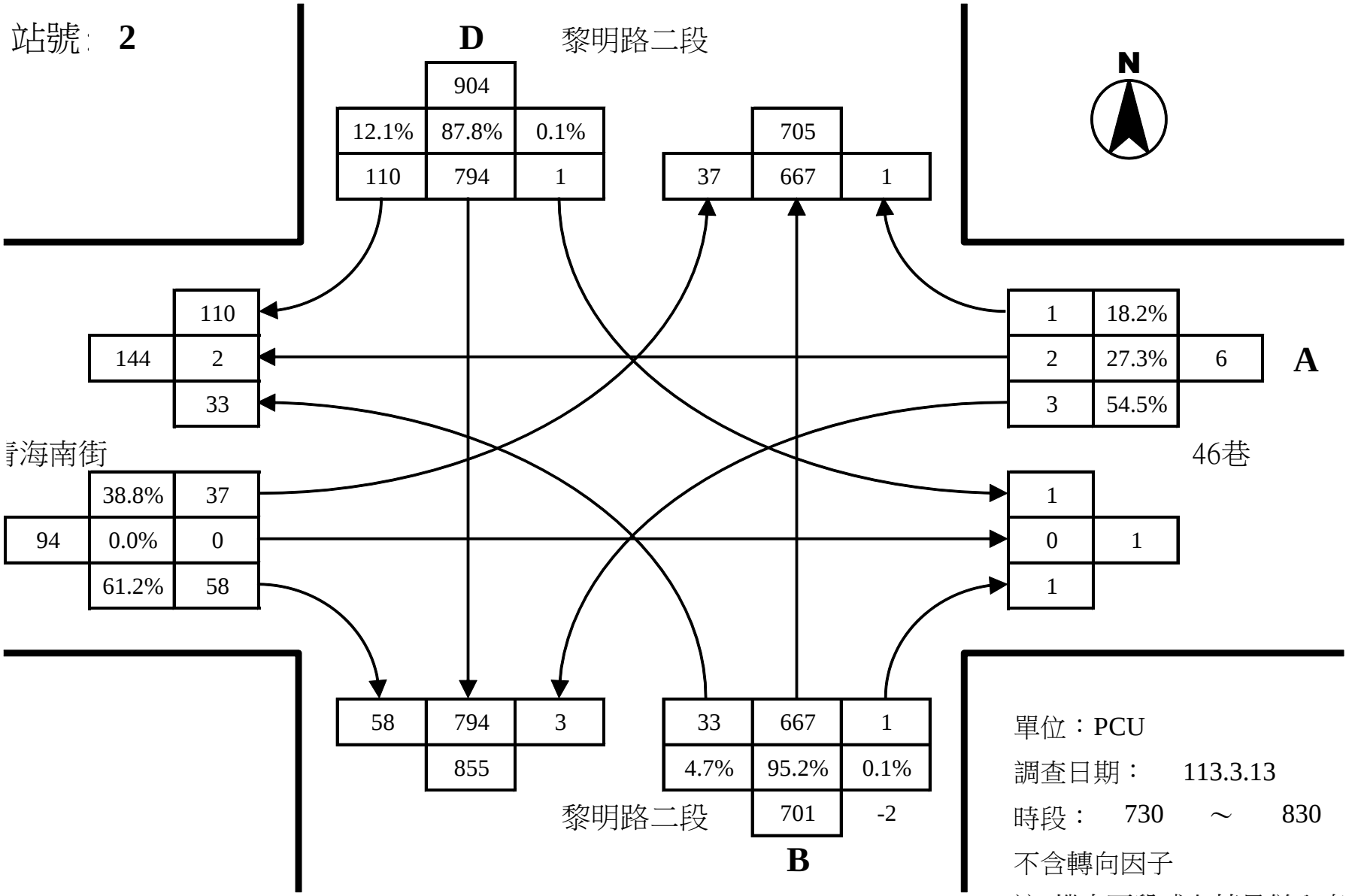
黎明路二段與青海南街路口平日晨峰轉向交通量示意圖
