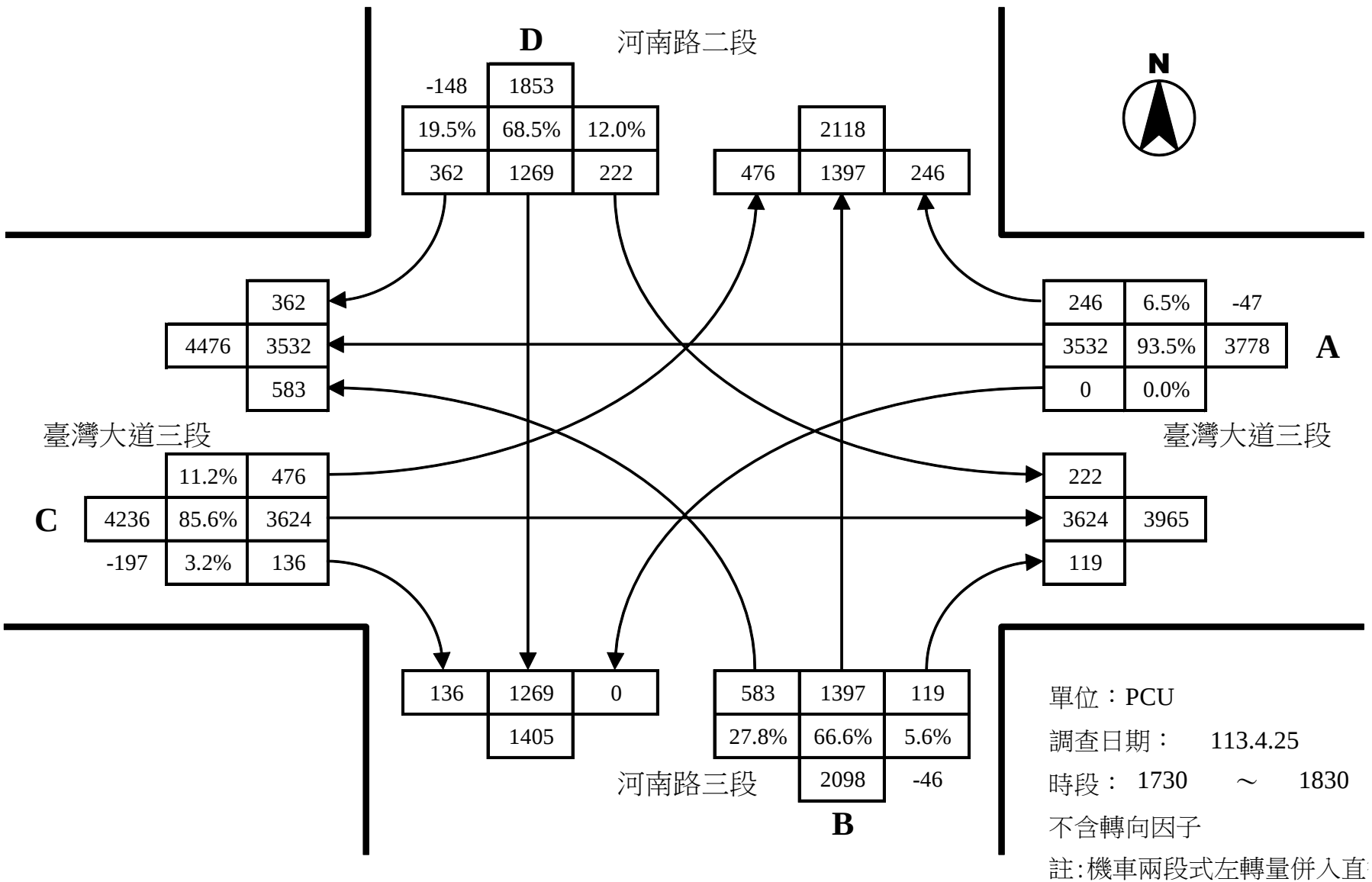
河南路二段與臺灣大道三段路口平日昏峰轉向交通量示意圖
