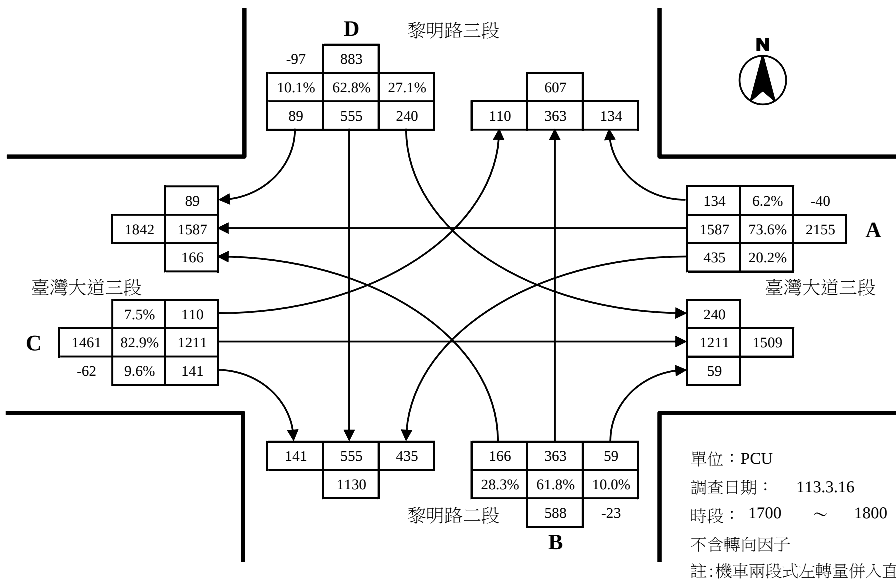
黎明路三段與臺灣大道三段路口假日尖峰轉向交通量示意圖
