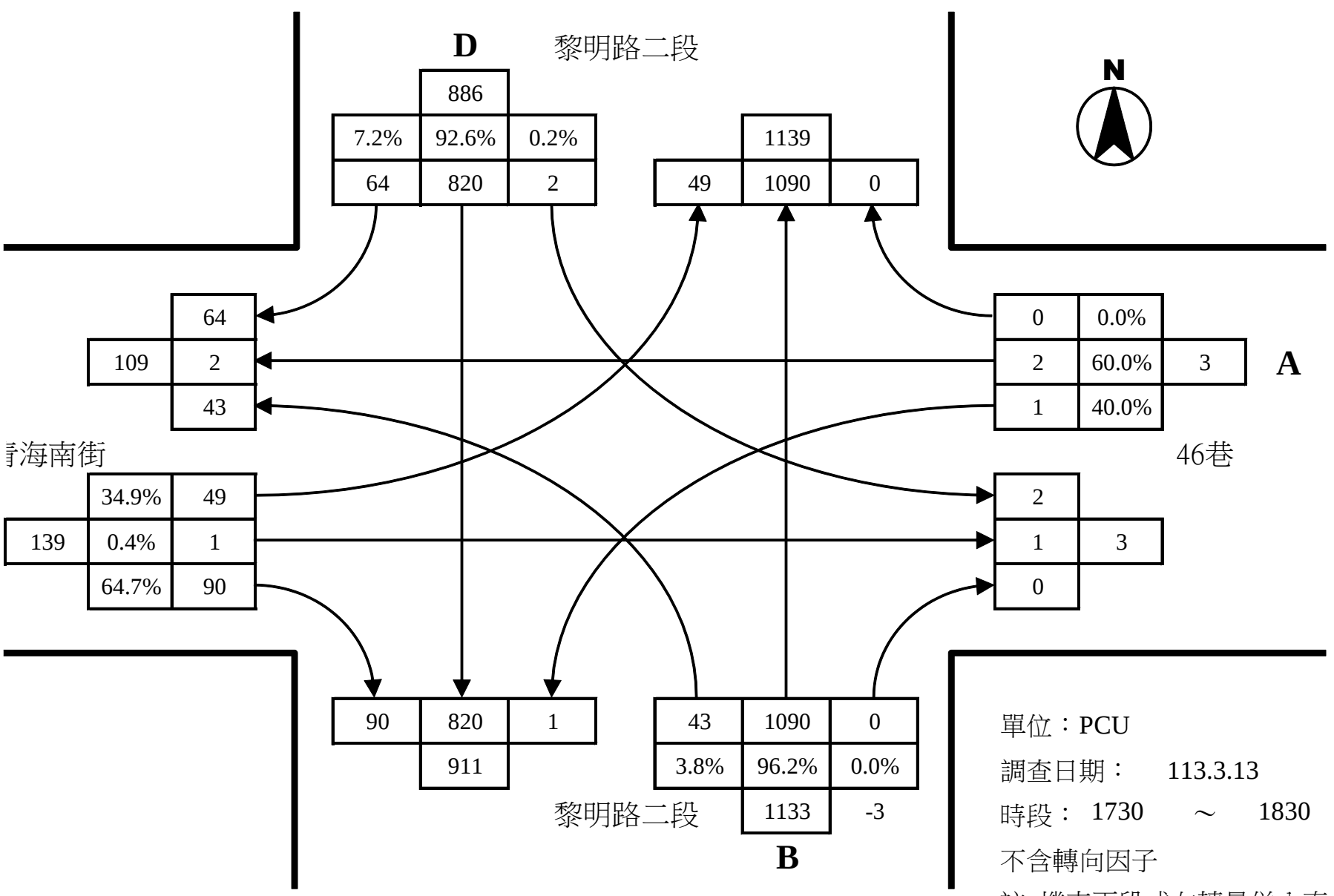
黎明路二段與青海南街路口平日昏峰轉向交通量示意圖
