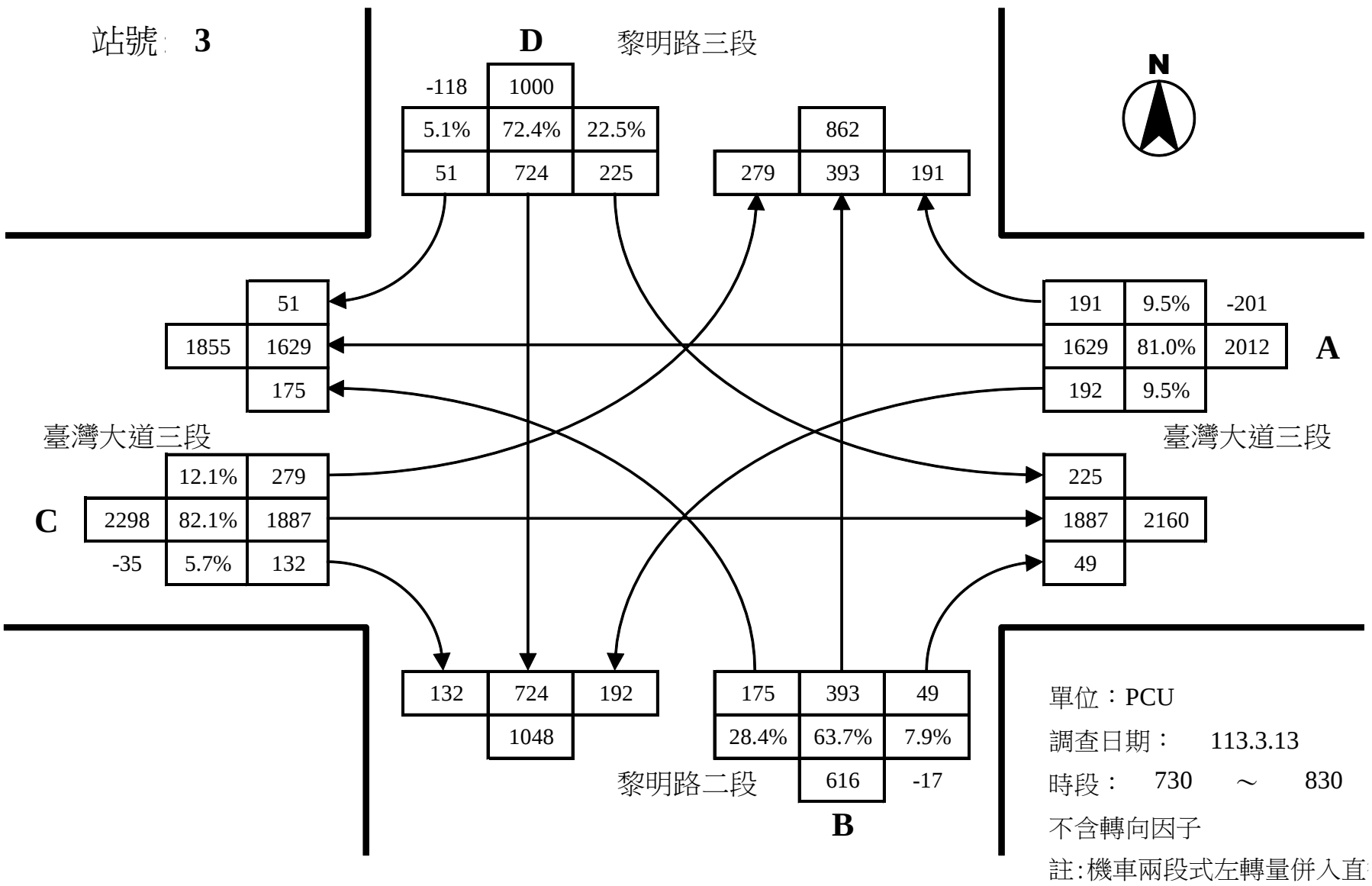
黎明路三段與臺灣大道三段路口平日晨峰轉向交通量示意圖
