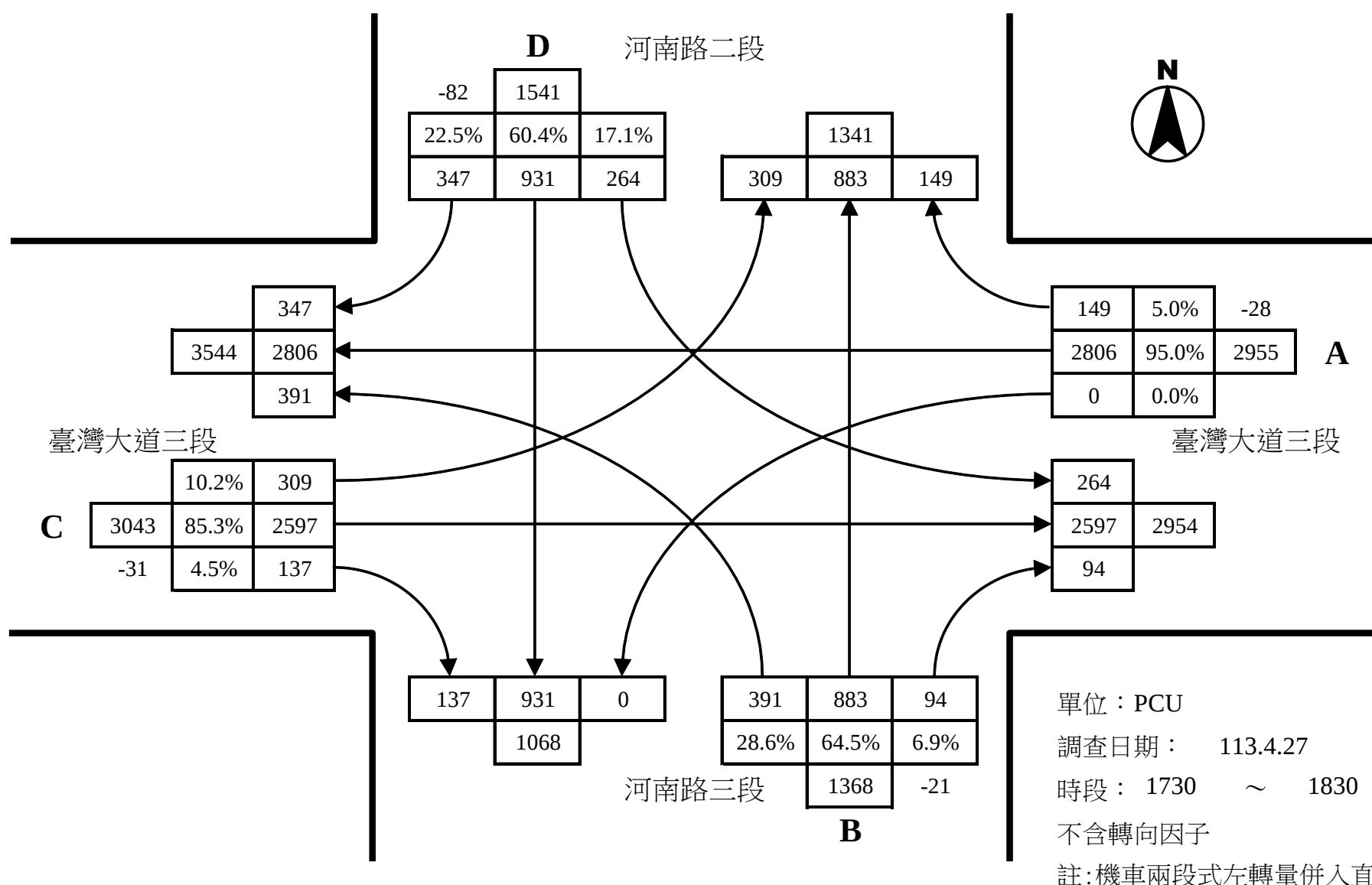
河南路二段與臺灣大道三段路口假日尖峰轉向交通量示意圖
