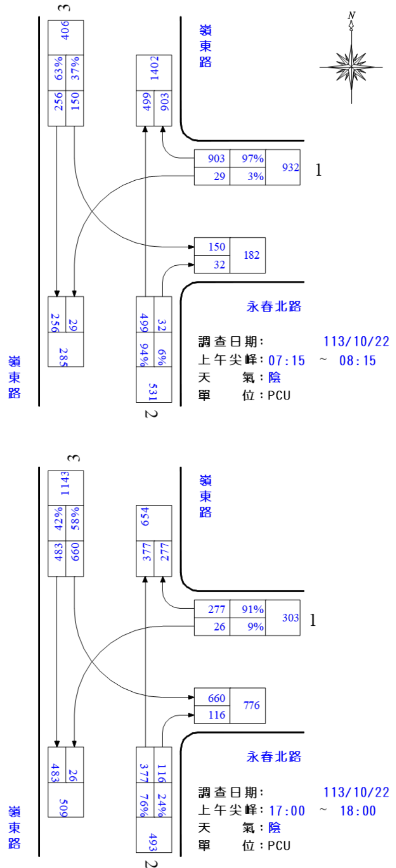
圖 1.1-5 永春北路/嶺東路平日晨昏峰路口轉向交通量示意圖
