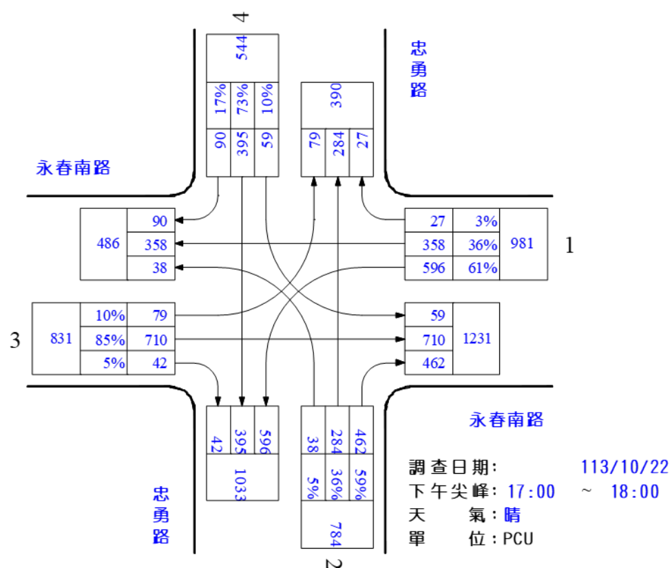
圖 1.1-4 永春南路/忠勇路平日晨昏峰路口轉向交通量示意圖
