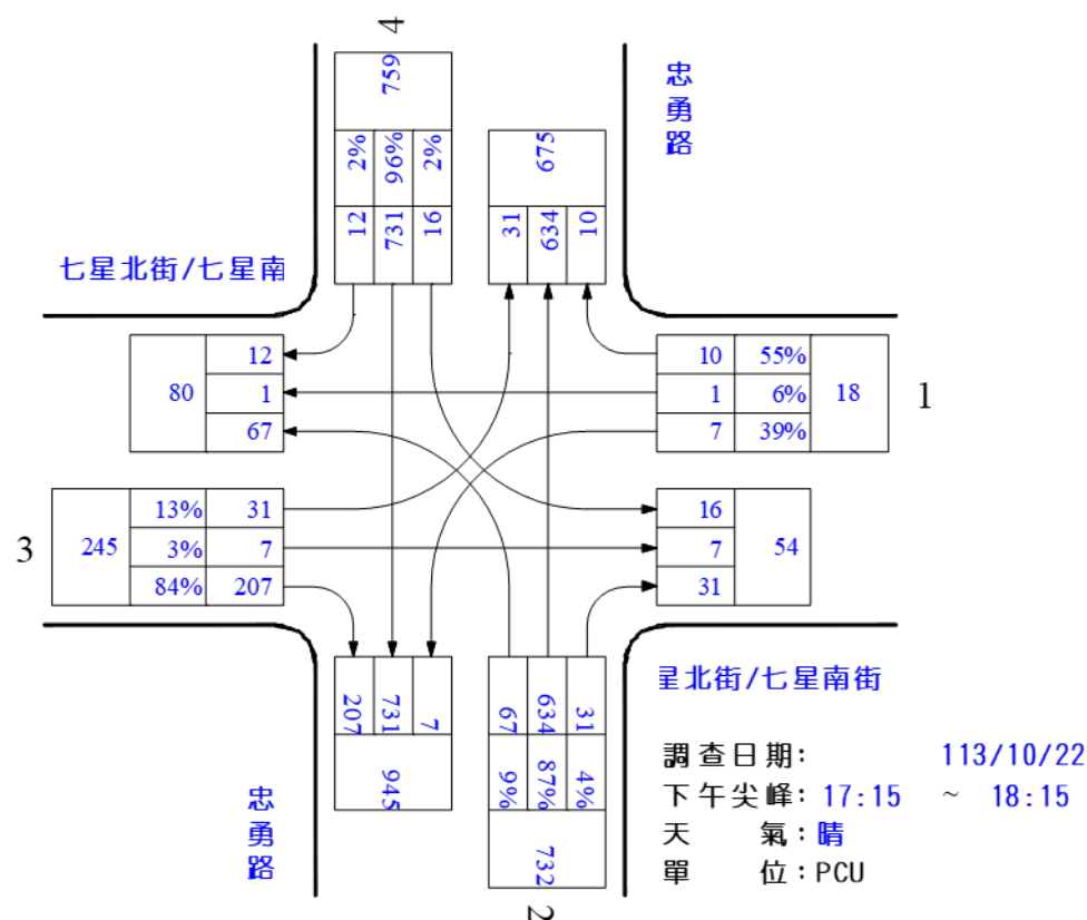
圖 1.1-2 七星北街/七星南街/忠勇路平日晨昏峰路口轉向交通量示意圖
