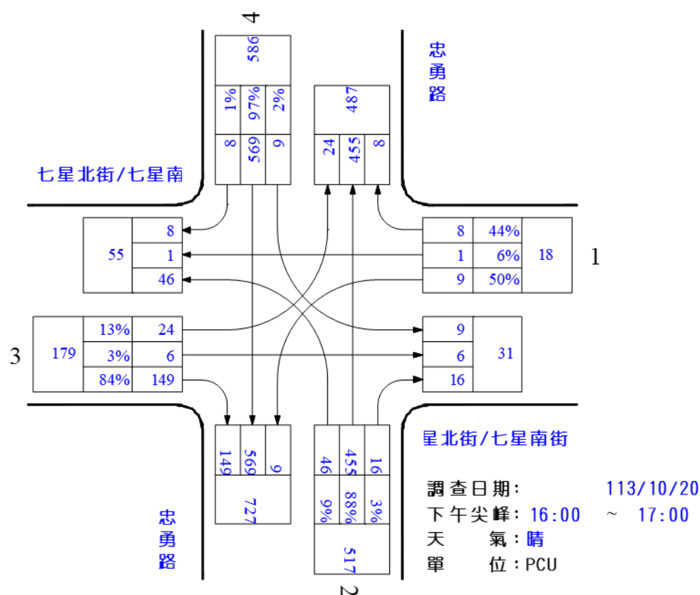
圖 1.1-6 七星北街/七星南街/忠勇路假日晨昏峰路口轉向交通量示意圖
