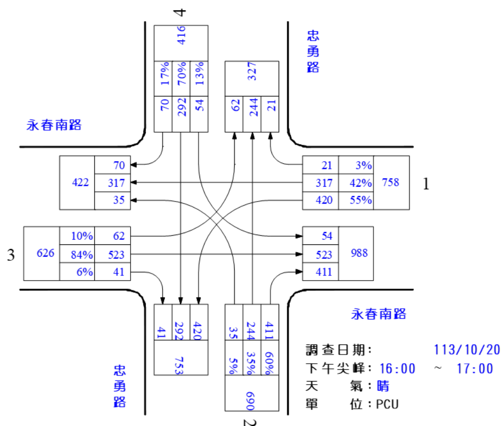
圖 1.1-8 永春南路/忠勇路假日晨昏峰路口轉向交通量示意圖
