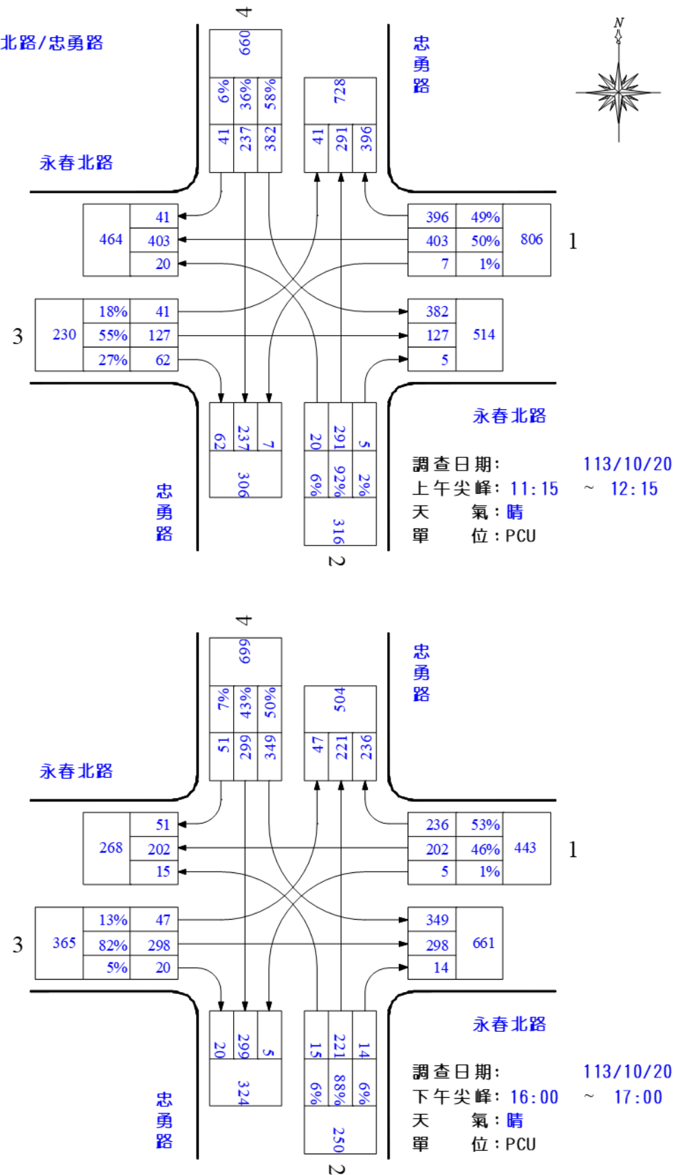
圖 1.1-7 永春北路/忠勇路假日晨昏峰路口轉向交通量示意圖
