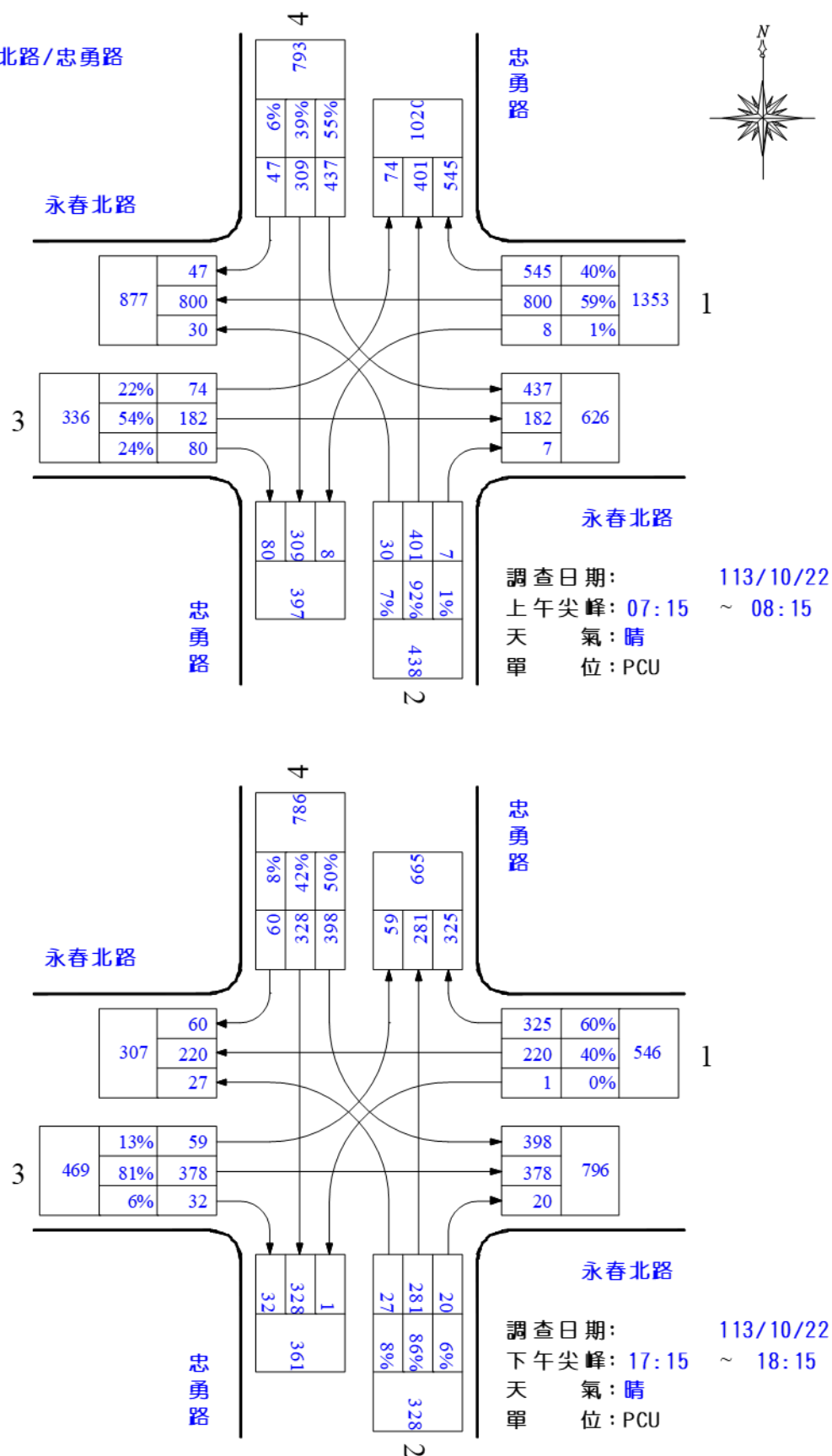
圖 1.1-3 永春北路/忠勇路平日晨昏峰路口轉向交通量示意圖
