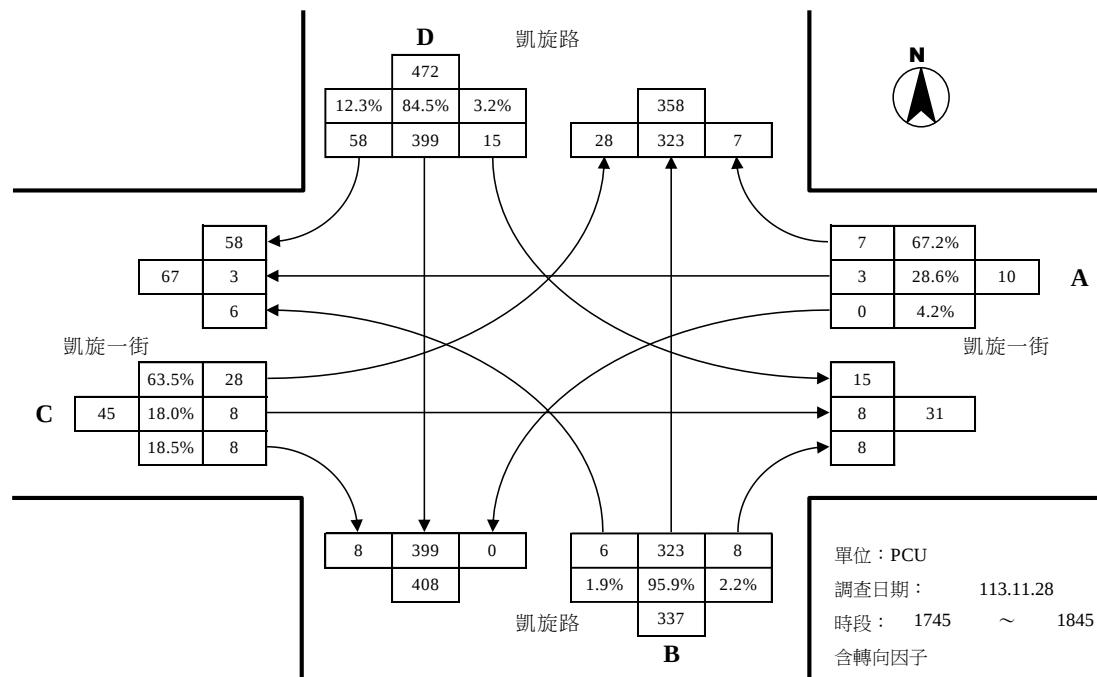
凱旋路與凱旋一街路口平日昏峰轉向交通量示意圖
