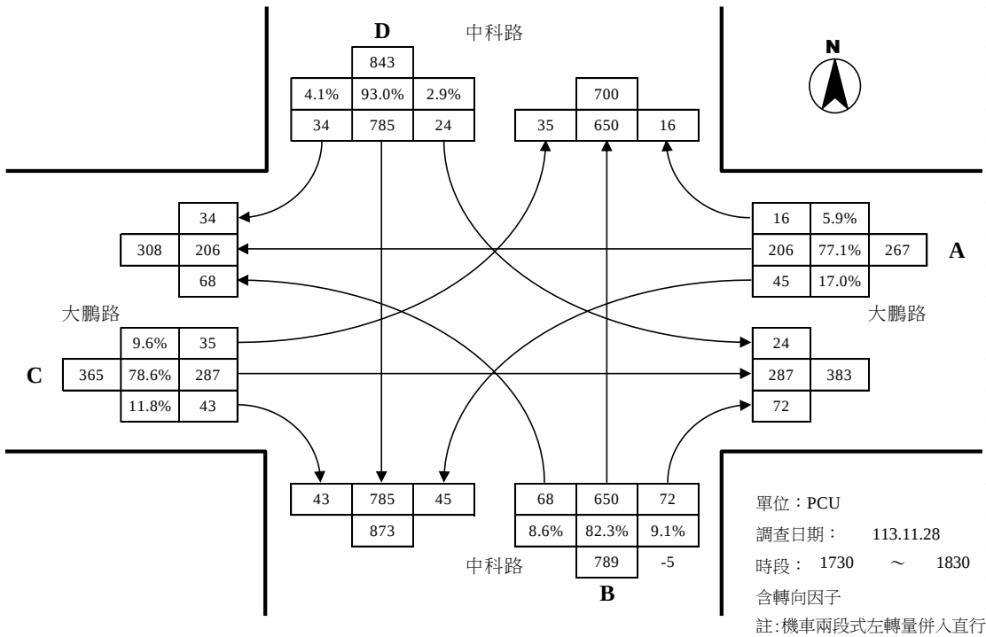
中科路與大鵬路路口平日昏峰轉向交通量示意圖
