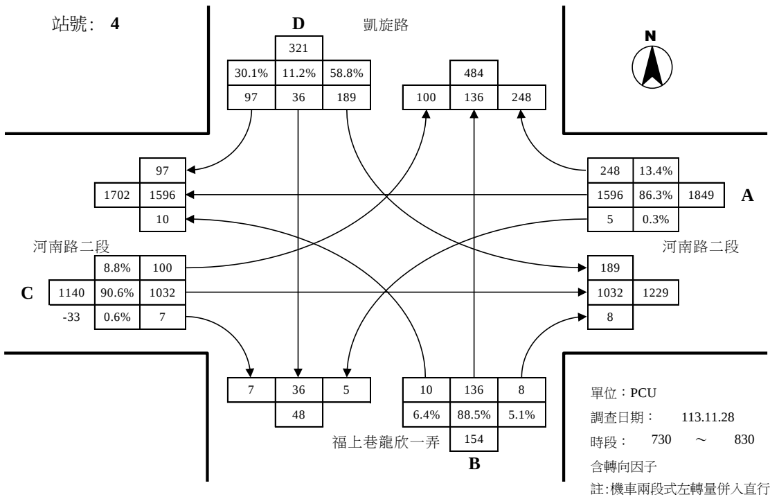
凱旋路與河南路二段路口平日晨峰轉向交通量示意圖
