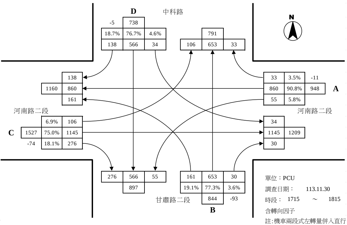
中科路與河南路二段路口假日尖峰轉向交通量示意圖
