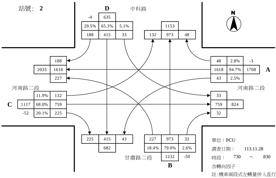
中科路與河南路二段路口平日晨峰轉向交通量示意圖
