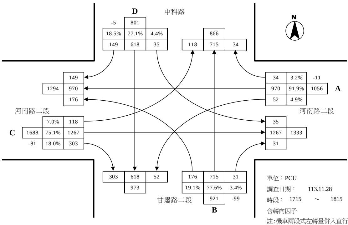
中科路與河南路二段路口平日昏峰轉向交通量示意圖
