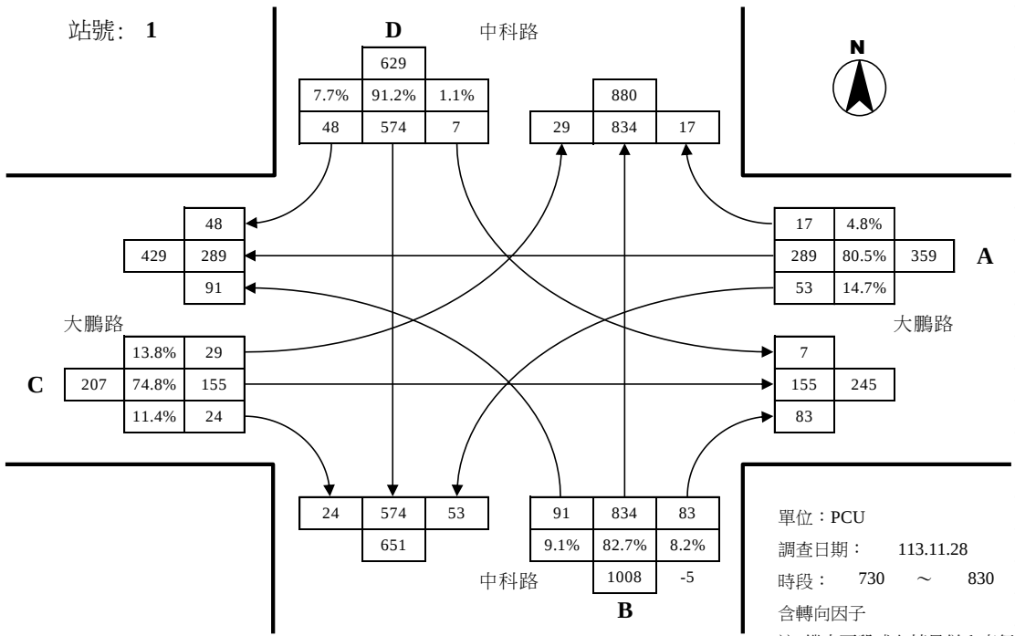
中科路與大鵬路路口平日晨峰轉向交通量示意圖
