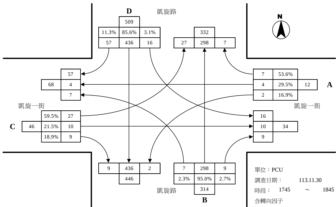
凱旋路與凱旋一街路口假日尖峰轉向交通量示意圖
