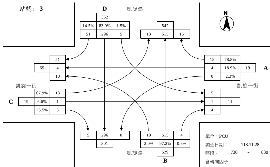
凱旋路與凱旋一街路口平日晨峰轉向交通量示意圖
