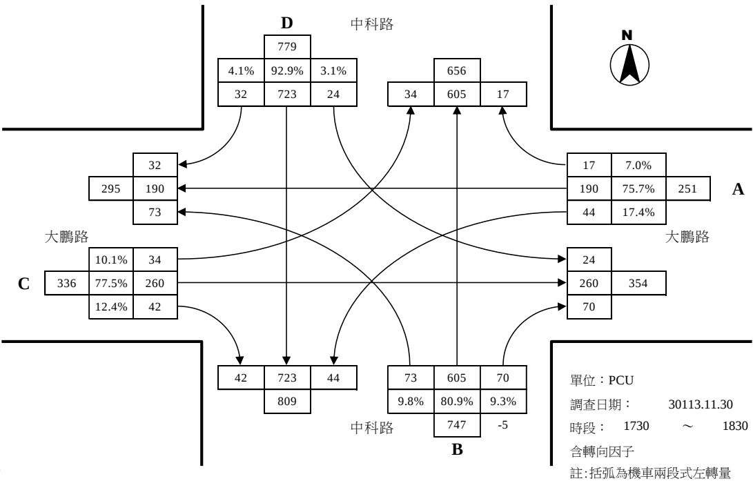
大鵬路與中科路路口假日尖峰轉向交通量示意圖
