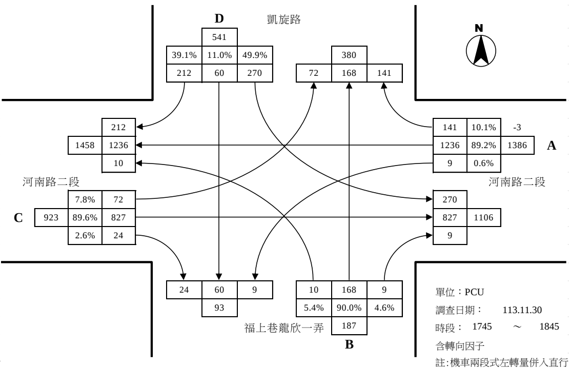
凱旋路與河南路二段路口假日尖峰轉向交通量示意圖
