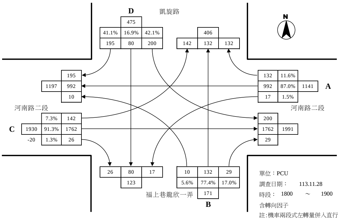
凱旋路與河南路二段路口平日昏峰轉向交通量示意圖
