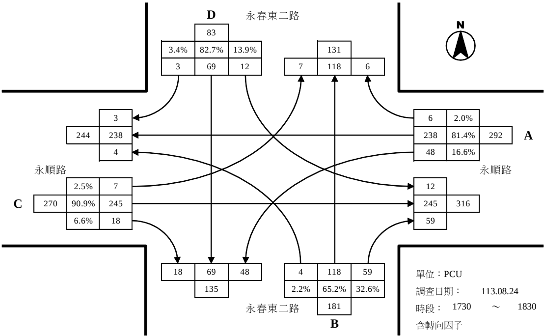
永順路與永春東二路路口假日尖峰轉向交通量示意圖
