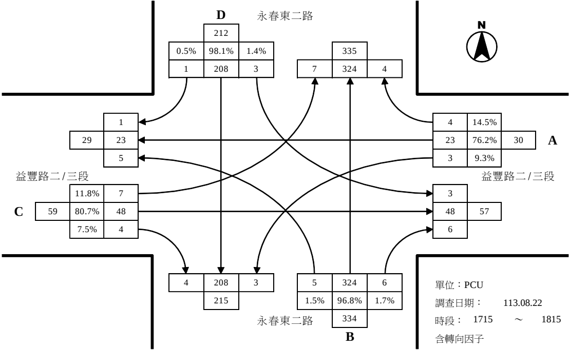
益豐路二/三段與永春東二路路口平日昏峰轉向交通量示意圖
