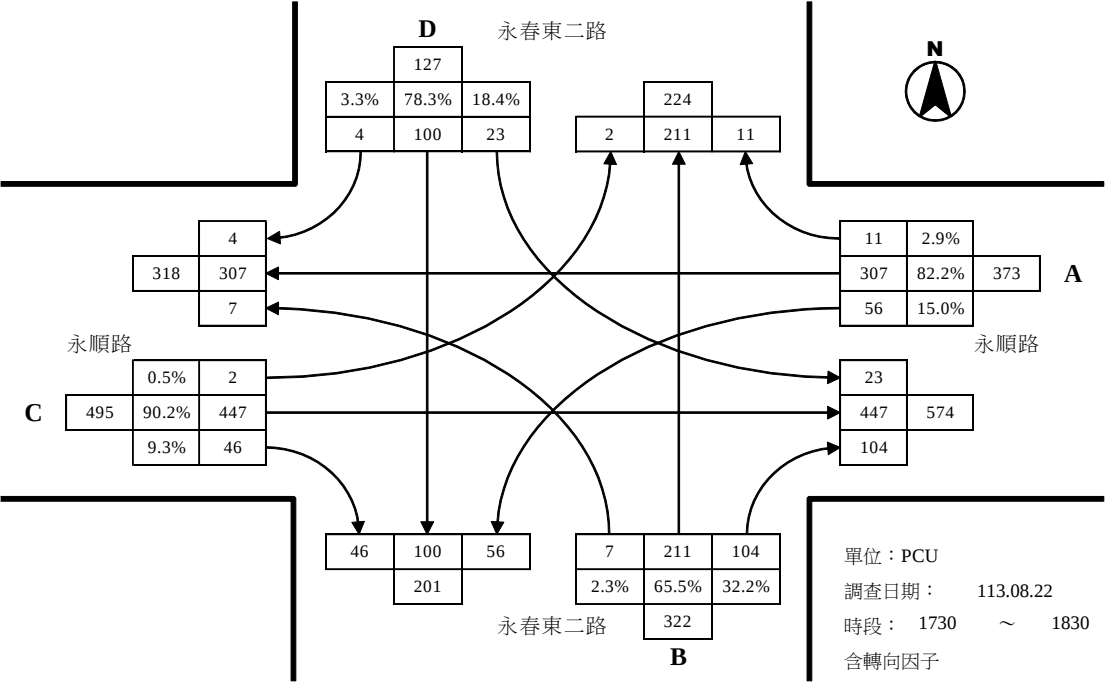
永順路與永春東二路路口平日昏峰轉向交通量示意圖
