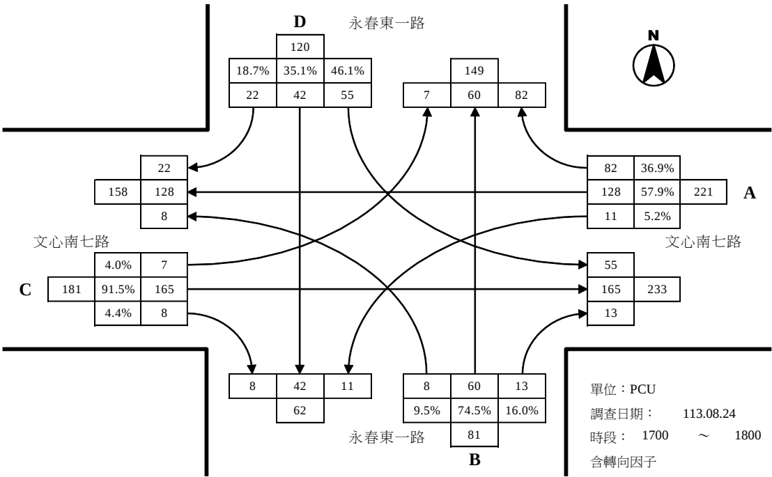
文心南七路與永春東一路路口假日尖峰轉向交通量示意圖
