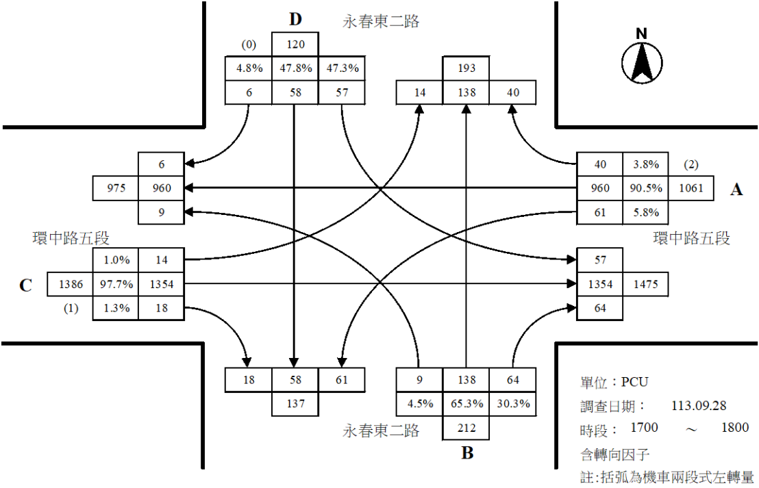
環中路五段與永春東二路路口假日尖峰轉向交通量示意圖
