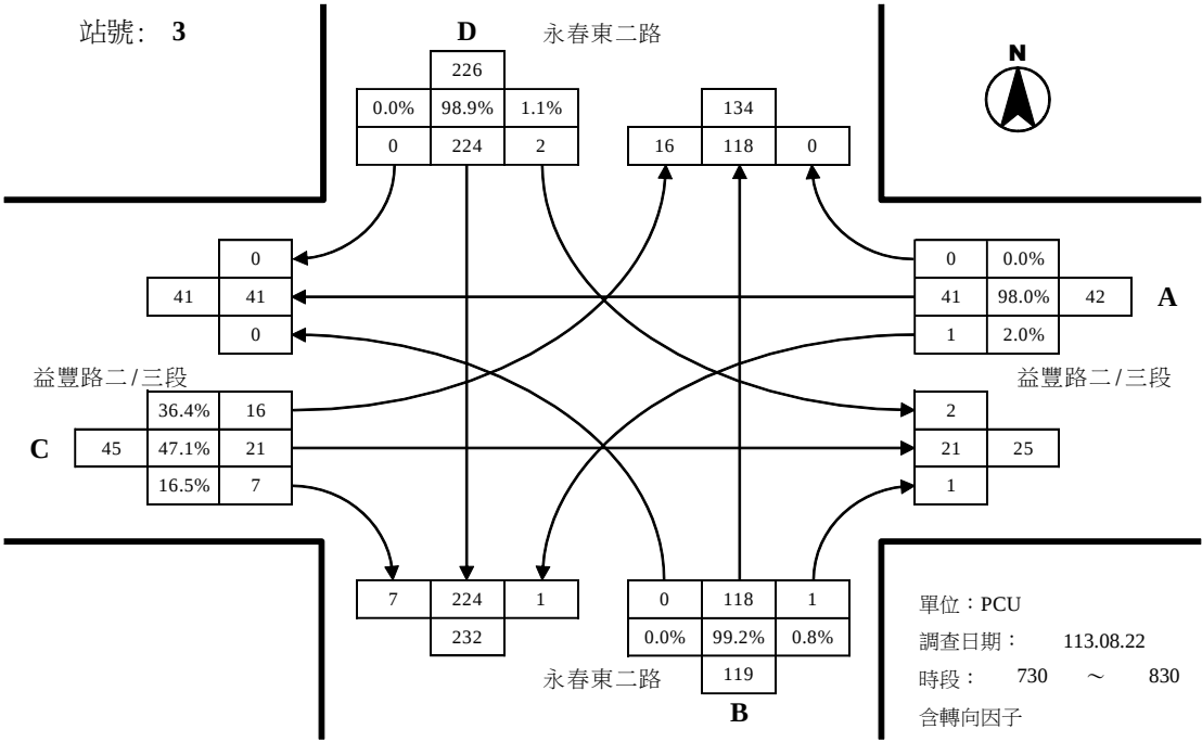
益豐路二/三段與永春東二路路口平日晨峰轉向交通量示意圖
