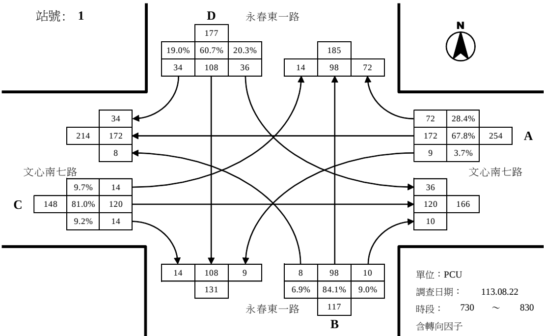
文心南七路與永春東一路路口平日晨峰轉向交通量示意圖
