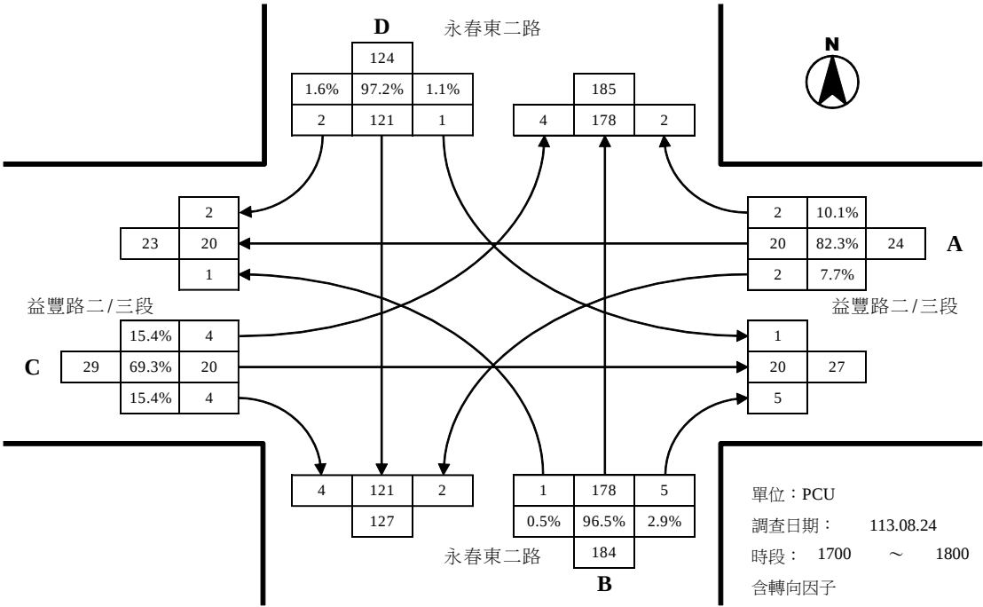
益豐路二/三段與永春東二路路口假日尖峰轉向交通量示意圖
