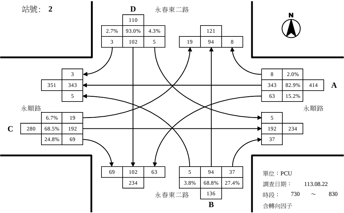
永順路與永春東二路路口平日晨峰轉向交通量示意圖
