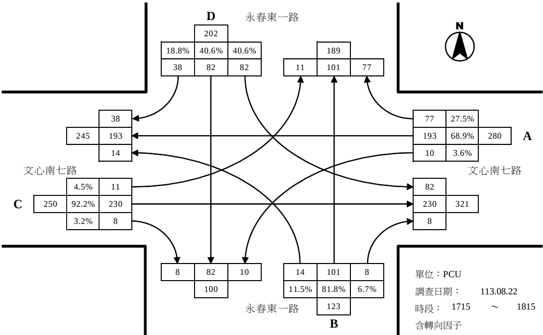
文心南七路與永春東一路路口平日昏峰轉向交通量示意圖
