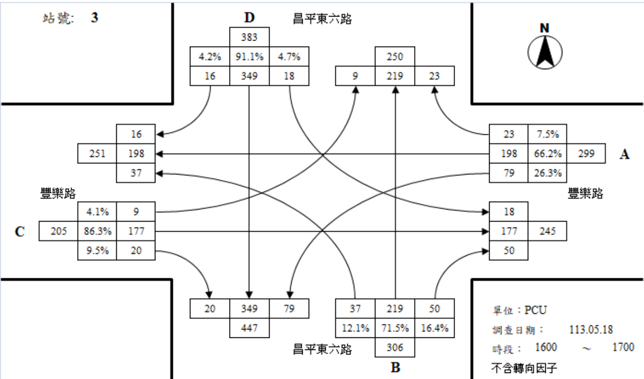
豐樂路與昌平東六路路口假日尖峰轉向交通量示意圖
