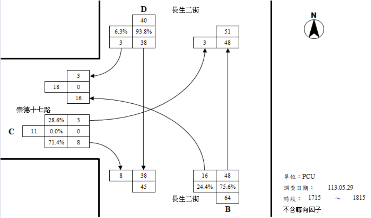
崇德十七路與長生二街路口平日昏峰轉向交通量示意圖
