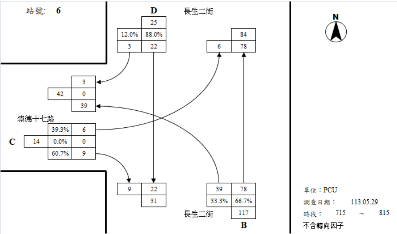
崇德十七路與長生二街路口平日晨峰轉向交通量示意圖
