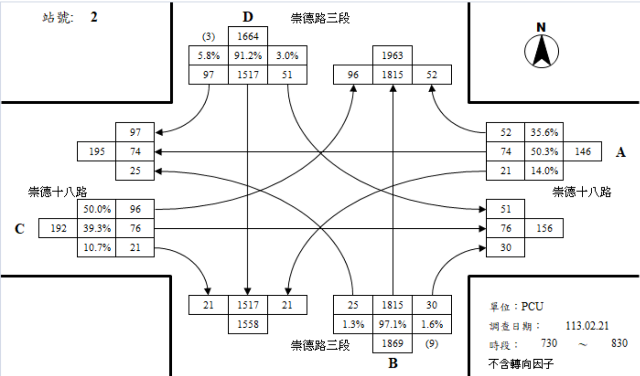
崇德十八路與崇德路三段路口平日晨峰轉向交通量示意圖
