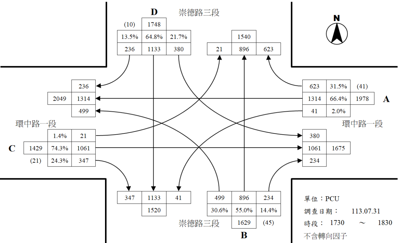
環中路一段與崇德路三段路口平日昏峰轉向交通量示意圖
