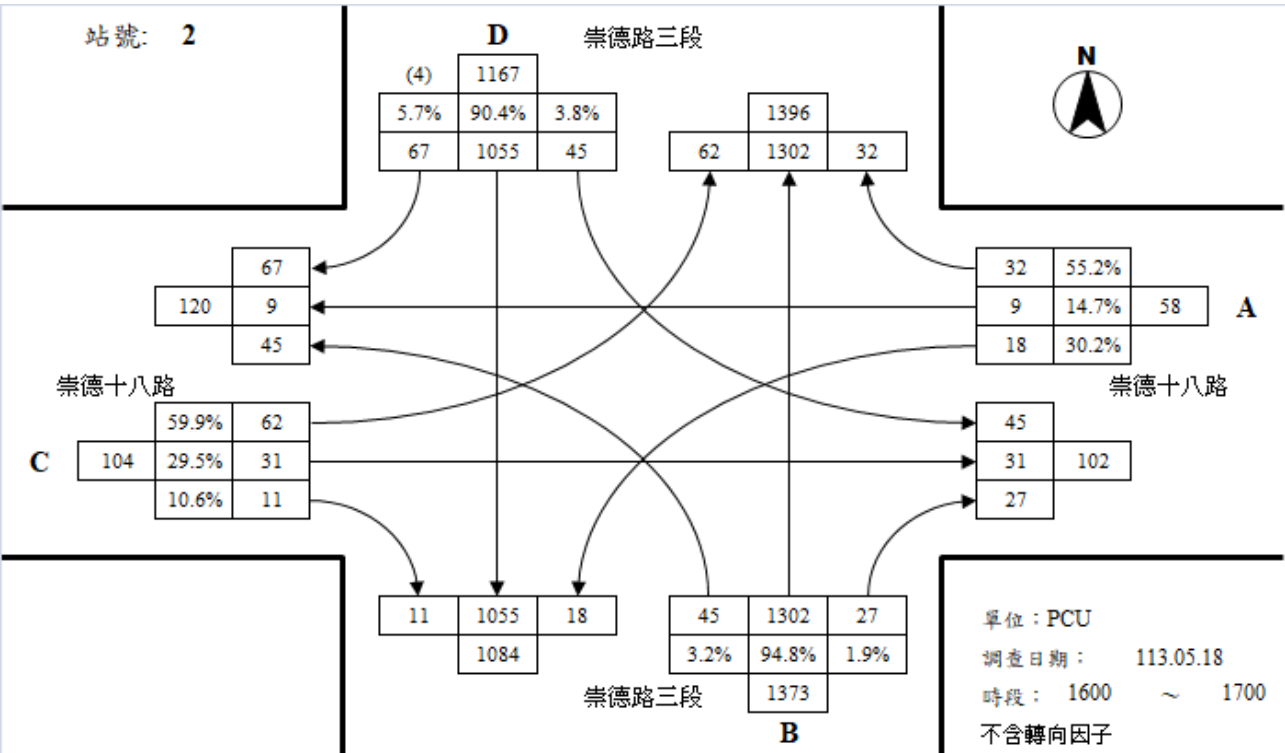
崇德十八路與崇德路三段路口假日尖峰轉向交通量示意圖
