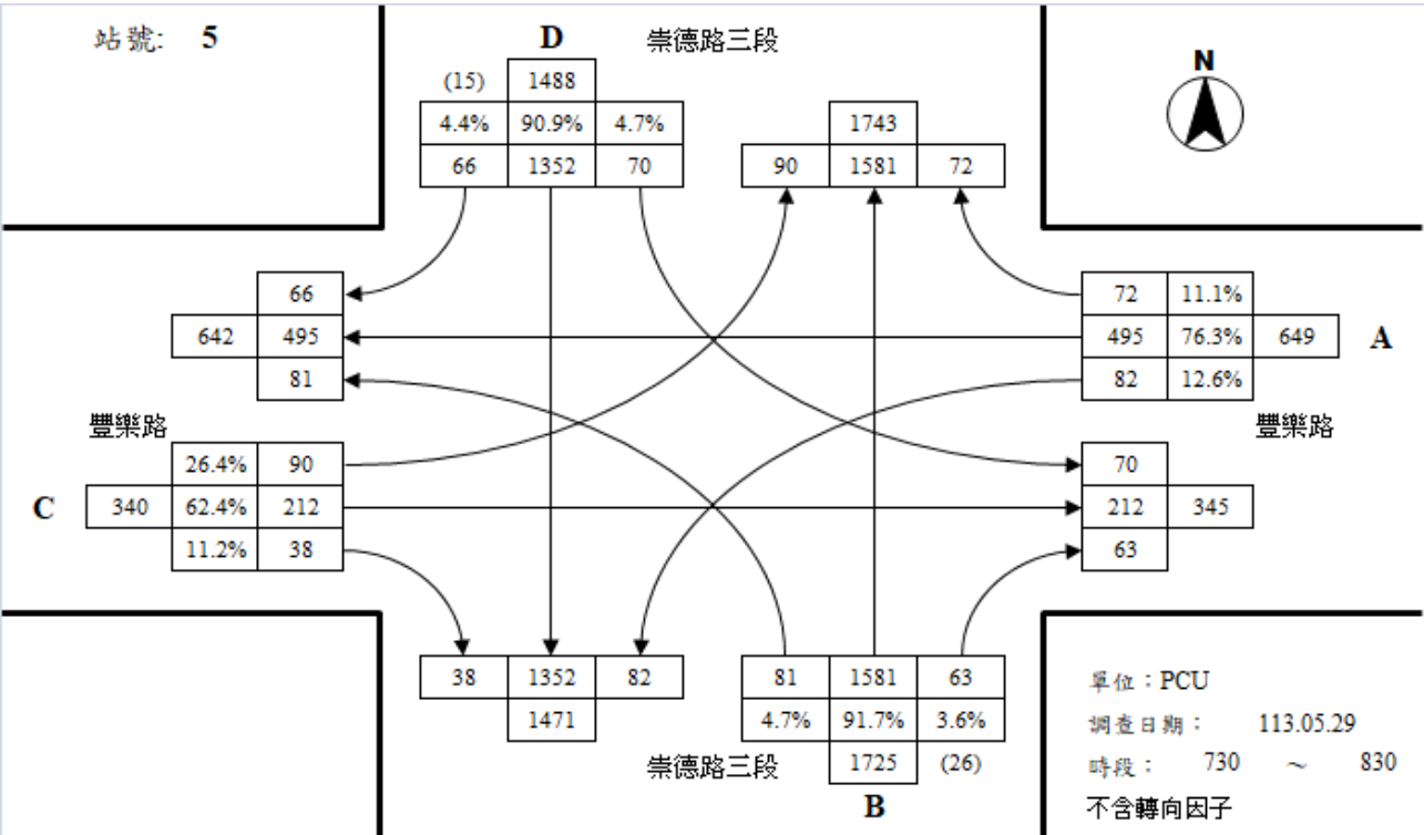
豐樂路與崇德路三段路口平日晨峰轉向交通量示意圖
