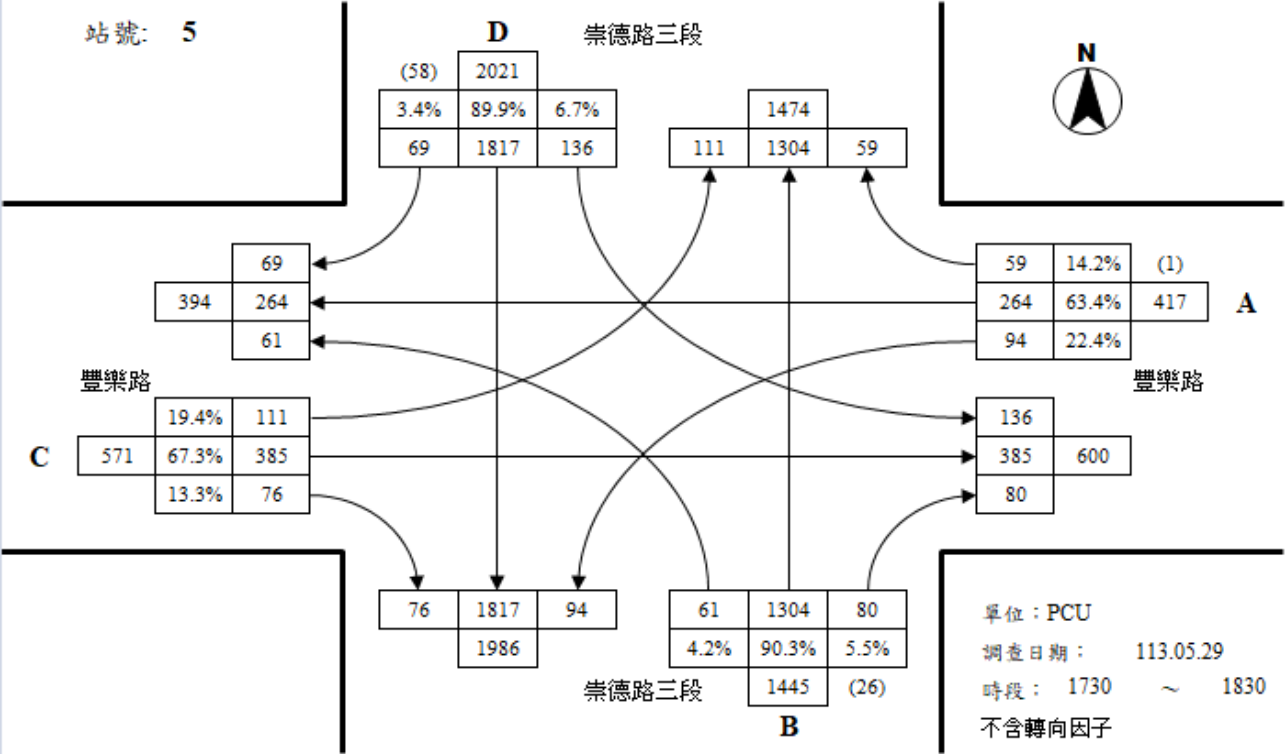
豐樂路與崇德路三段路口假日尖峰轉向交通量示意圖
