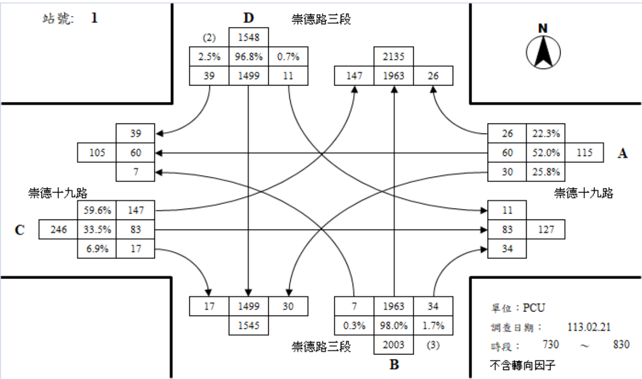
崇德十九路與崇德路三段路口平日晨峰轉向交通量示意圖
