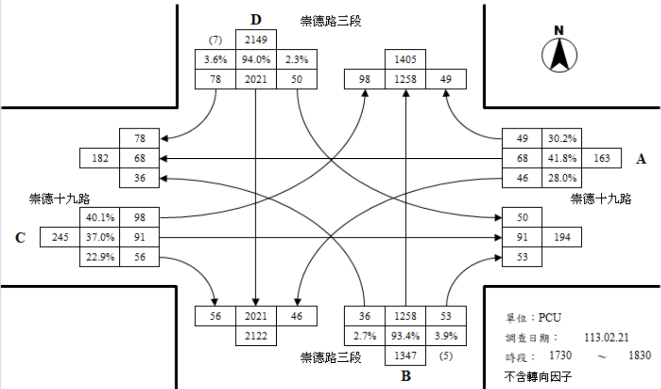
崇德十九路與崇德路三段路口平日昏峰轉向交通量示意圖
