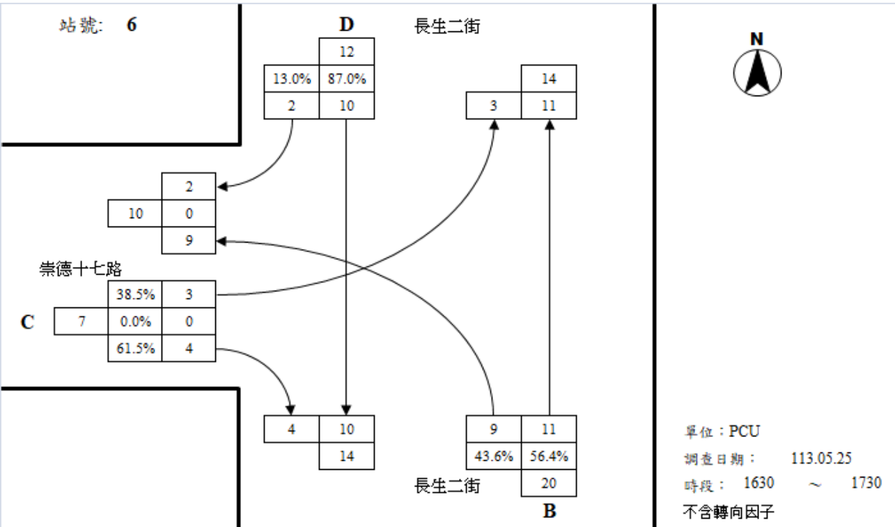
崇德十七路與長生二街路口假日尖峰轉向交通量示意圖
