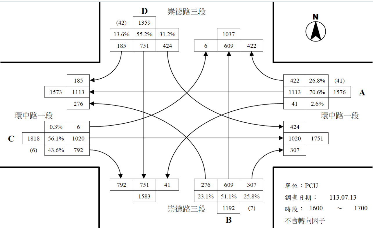
環中路一段與崇德路三段路口假日賽前轉向交通量示意圖
