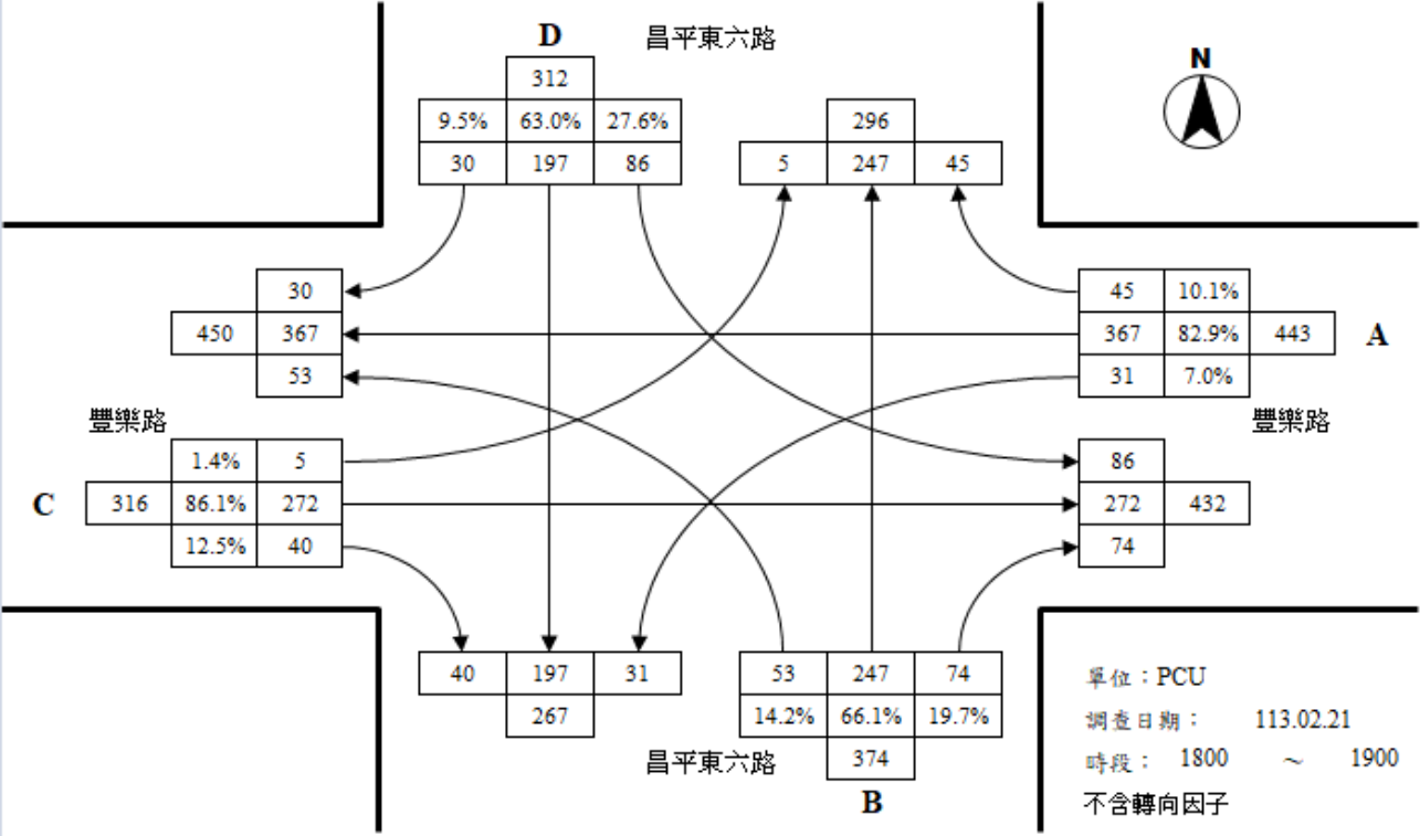
豐樂路與昌平東六路路口平日昏峰轉向交通量示意圖
