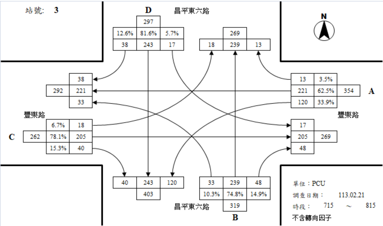
豐樂路與昌平東六路路口平日晨峰轉向交通量示意圖
