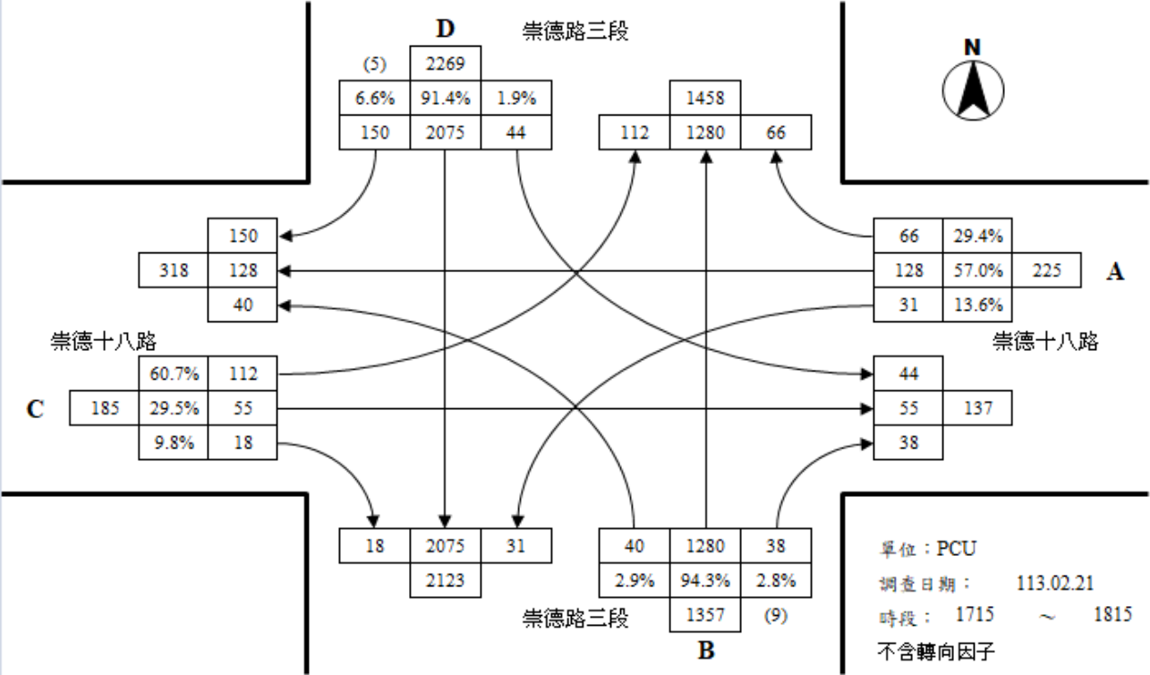
崇德十八路與崇德路三段路口平日昏峰轉向交通量示意圖
