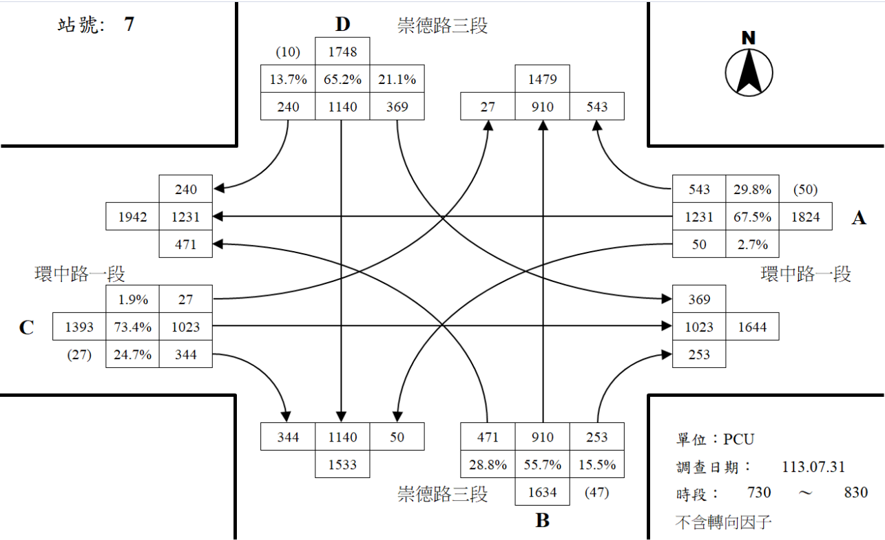
環中路一段與崇德路三段路口平日晨峰轉向交通量示意圖
