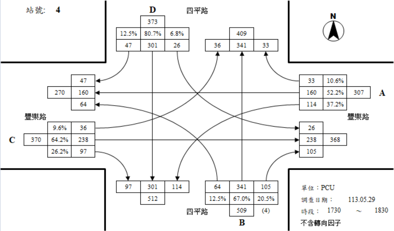
豐樂路與四平路路口假日尖峰轉向交通量示意圖
