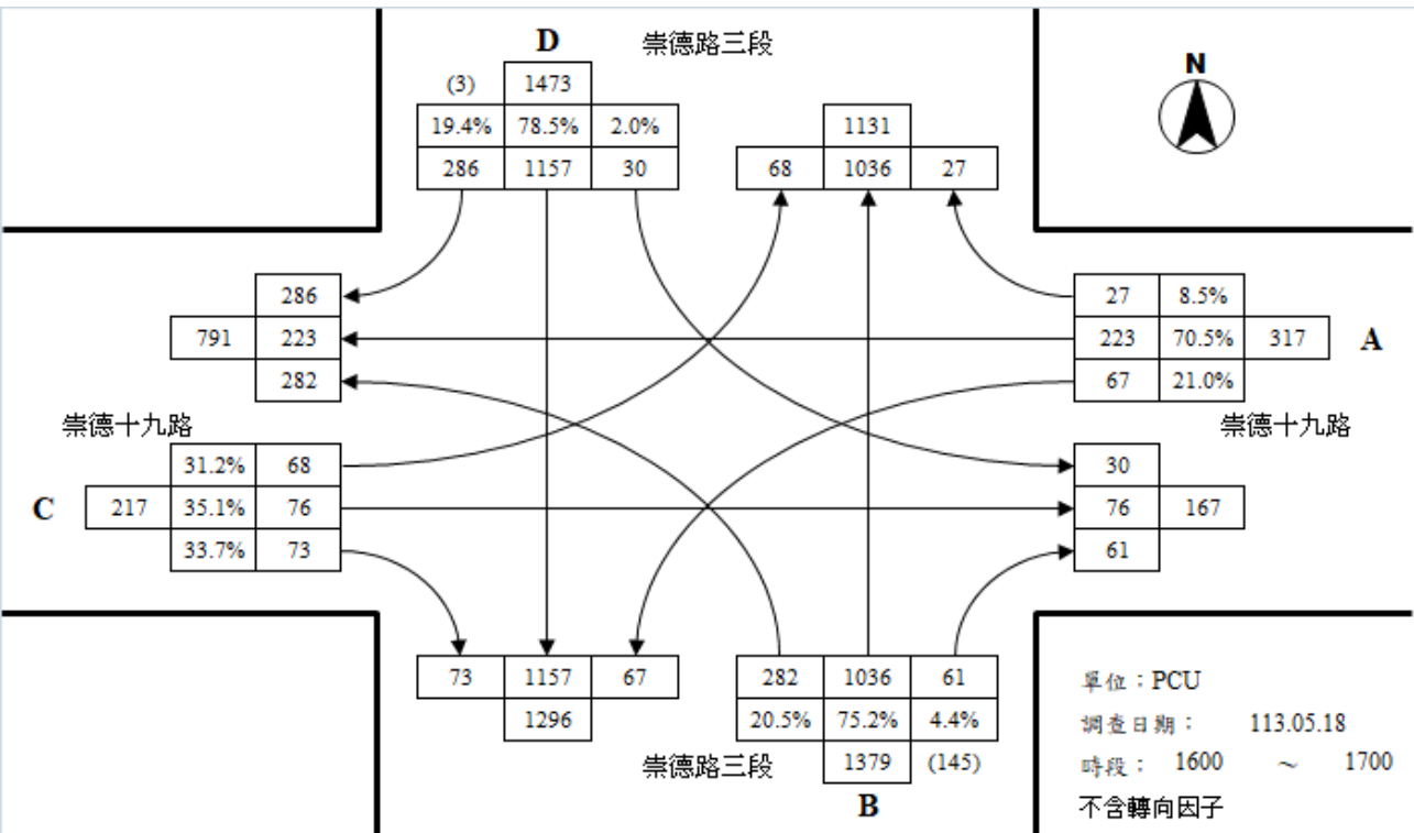
崇德十九路與崇德路三段路口假日賽前轉向交通量示意圖
