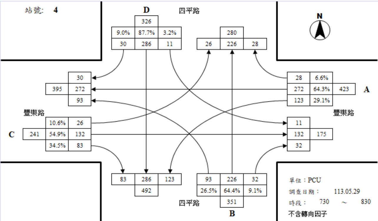
豐樂路與四平路路口平日晨峰轉向交通量示意圖
