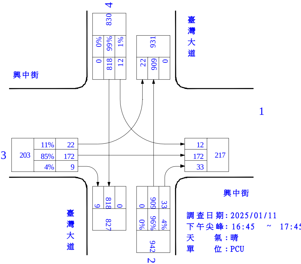
圖 1.1-8 臺灣大道/興中街路口轉向交通量示意圖(假日)
