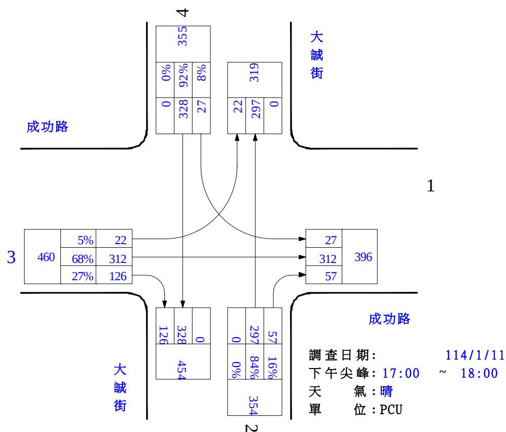
圖 1.1-9 大誠街/成功路路口轉向交通量示意圖(假日)
