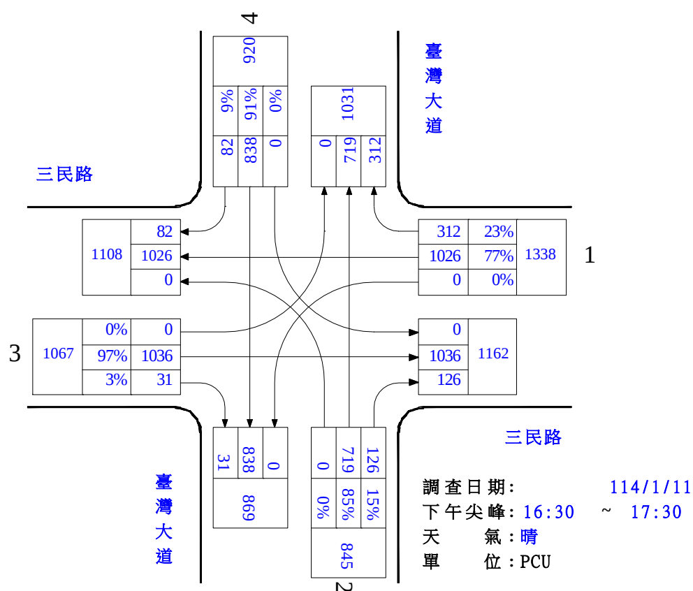
圖 1.1-11 臺灣大道/三民路路口轉向交通量示意圖(假日)
