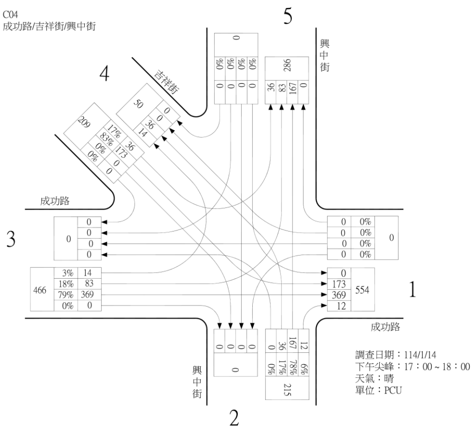
圖 1.1-5 成功路/吉祥街/興中街路口轉向交通量示意圖(平日)
