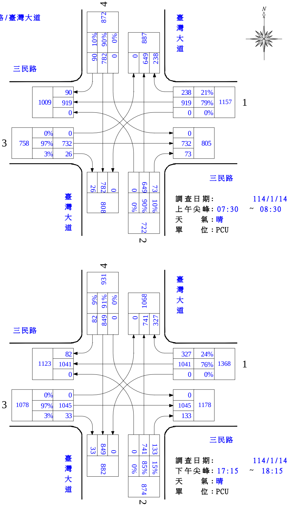
圖 1.1-6 臺灣大道/三民路路口轉向交通量示意圖(平日)
