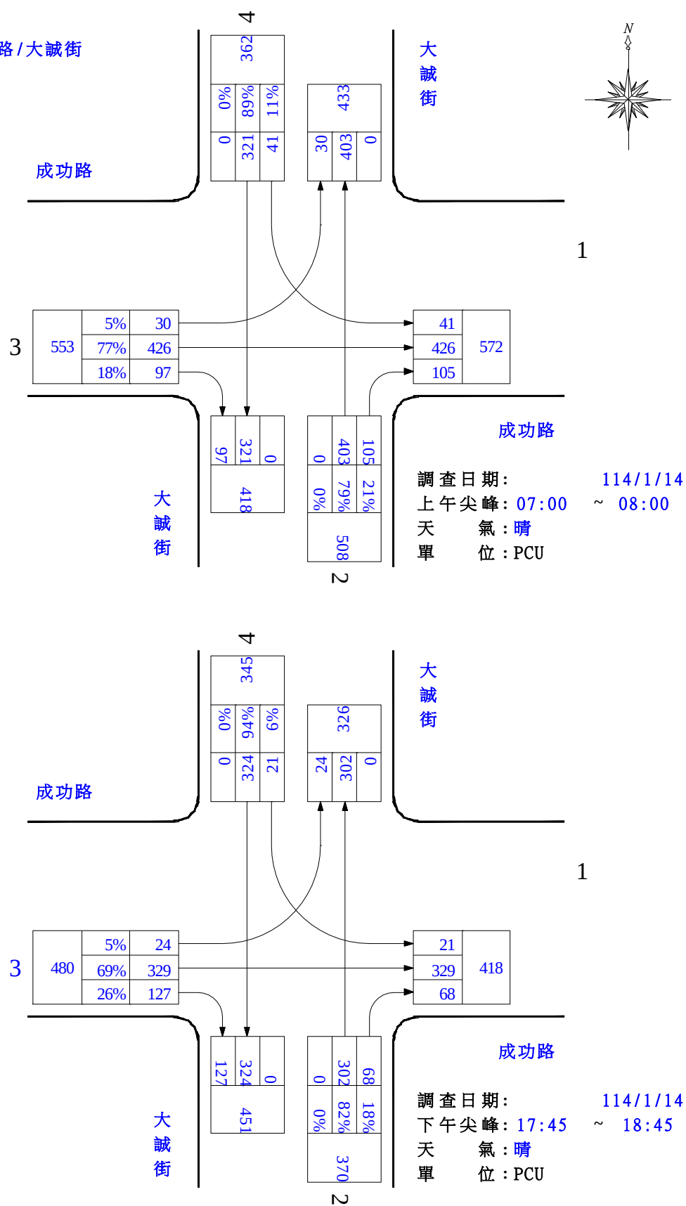
圖 1.1-4 大誠街/成功路路口轉向交通量示意圖(平日)
