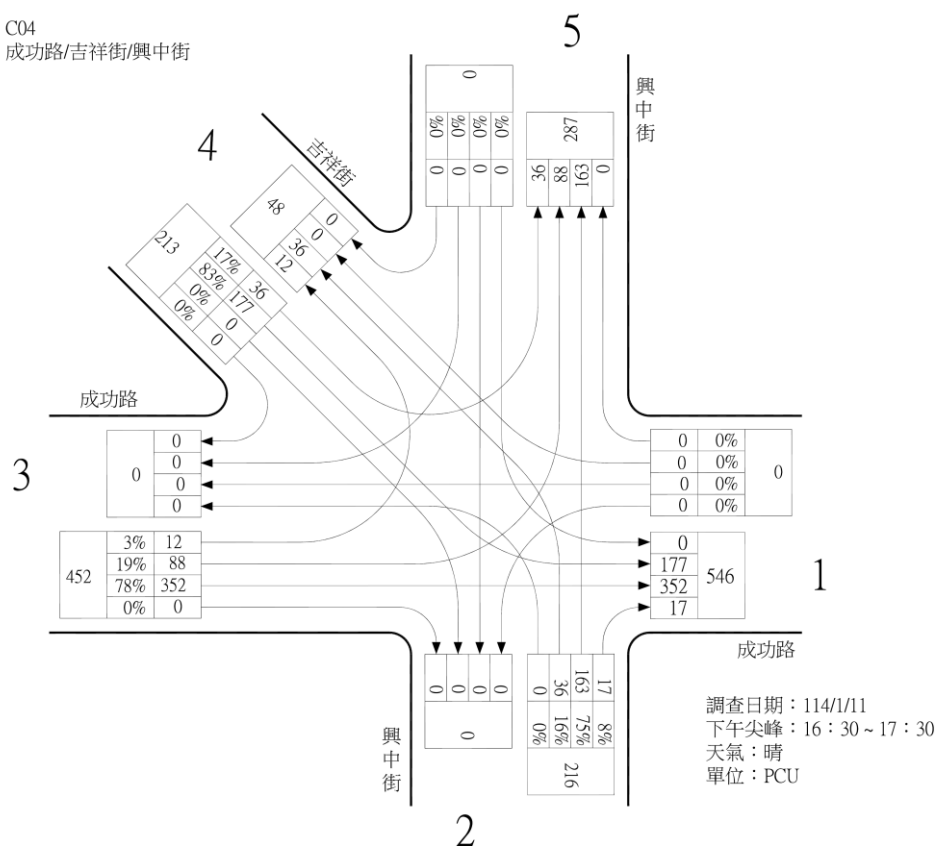
圖 1.1-10 成功路/吉祥街/興中街路口轉向交通量示意圖(假日)
