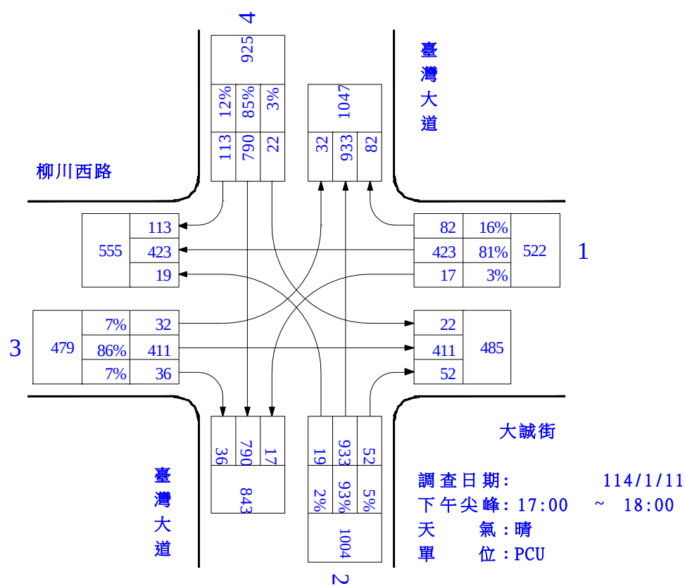
圖 1.1-7 臺灣大道/大誠街/柳川西路路口轉向交通量示意圖(假日)
