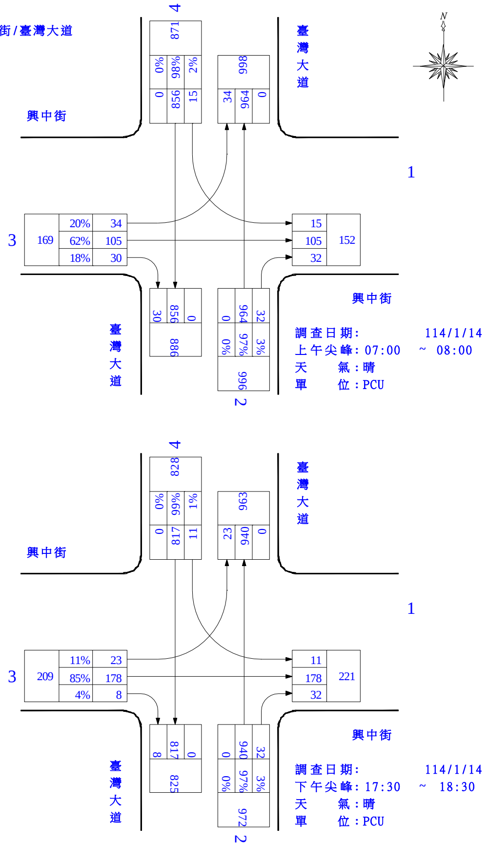
圖 1.1-3 臺灣大道/興中街路口轉向交通量示意圖(平日)
