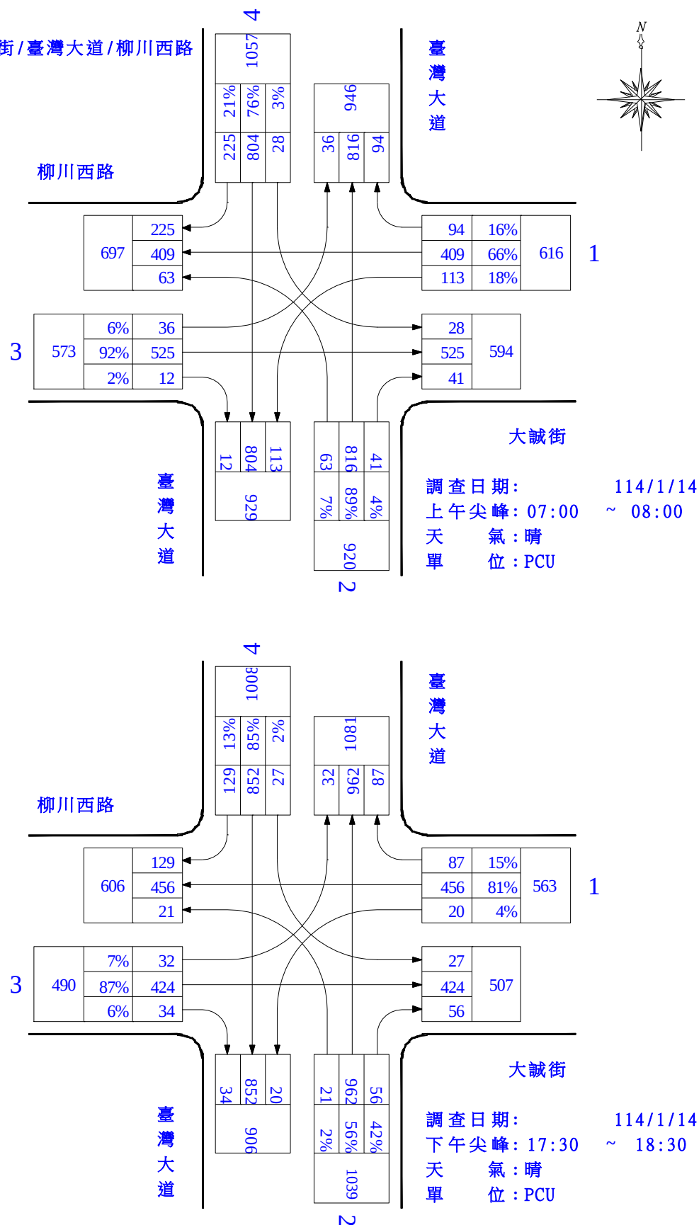
圖 1.1-2 臺灣大道/大誠街/柳川西路路口轉向交通量示意圖(平日)
