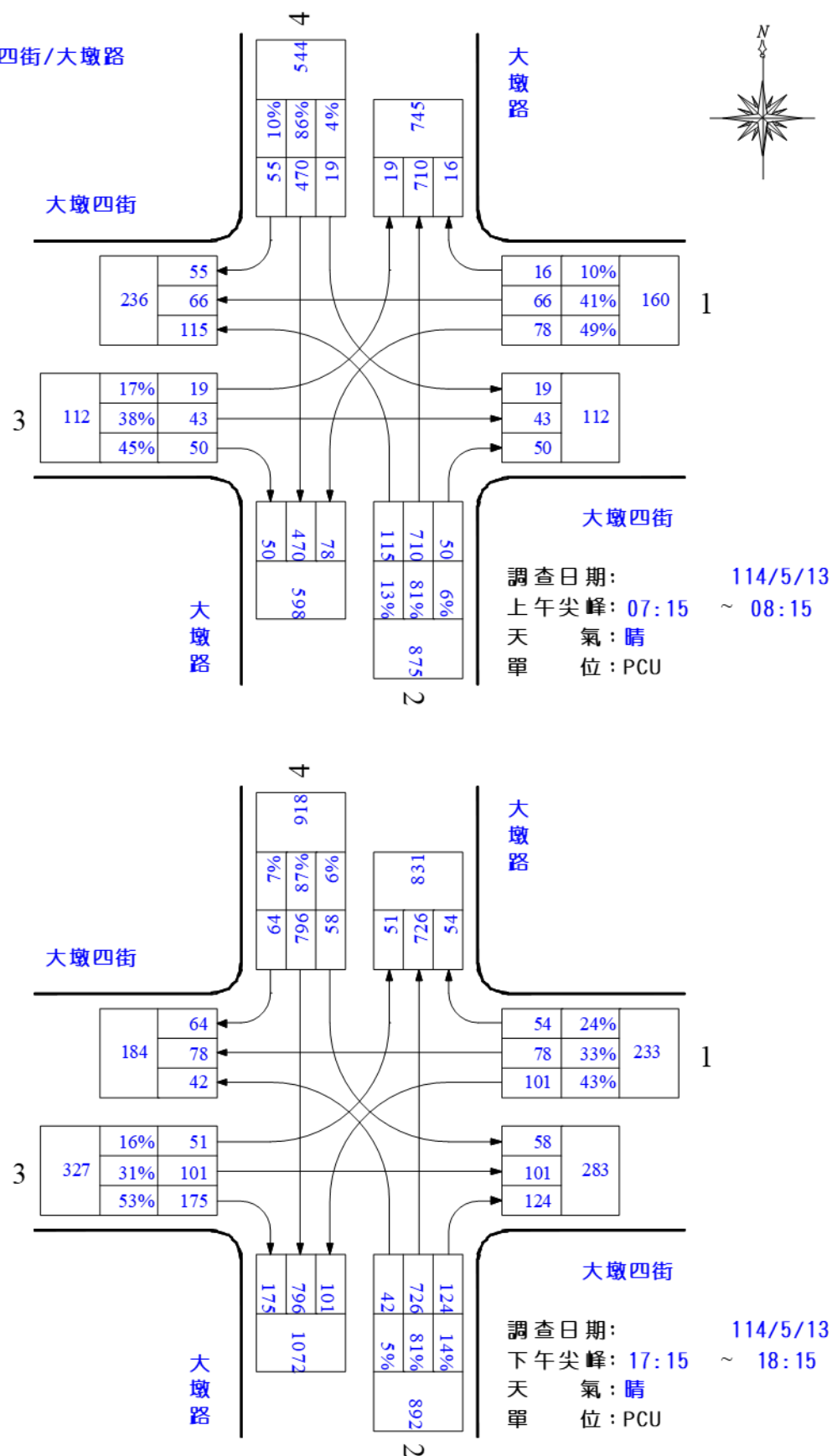
圖 1.1-5 大墩四街/大墩路平日晨昏峰路口轉向交通量示意圖
