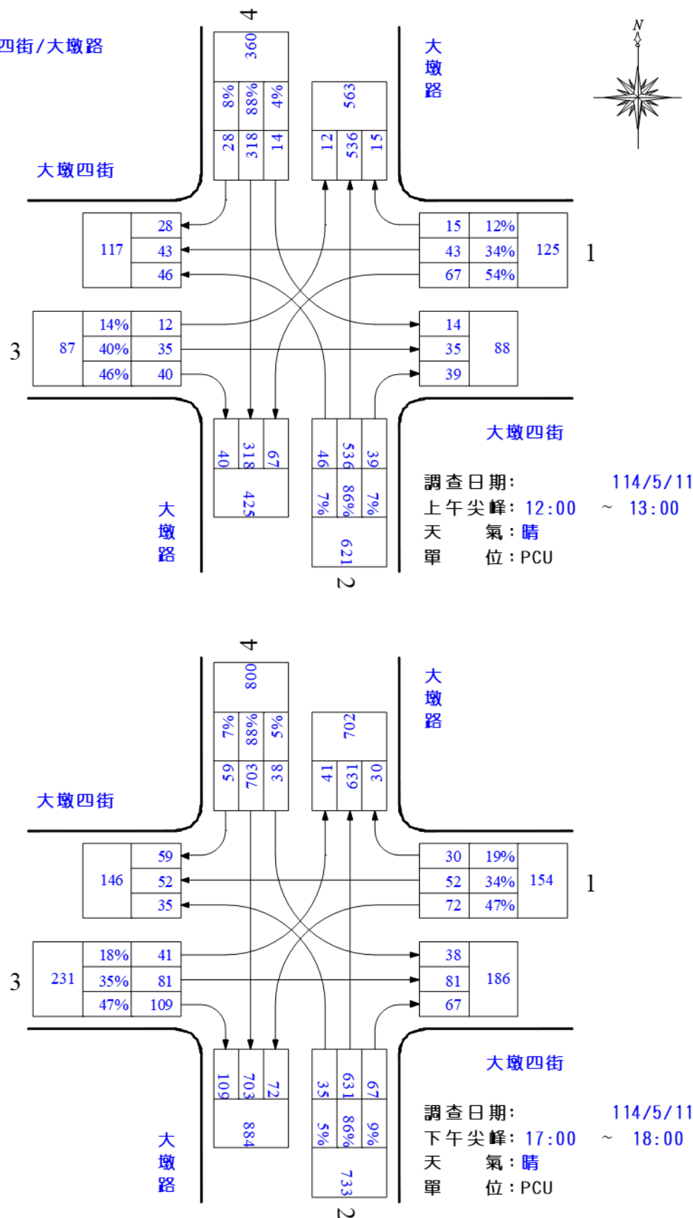
圖 1.1-10 大墩四街/大墩路假日晨昏峰路口轉向交通量示意圖
