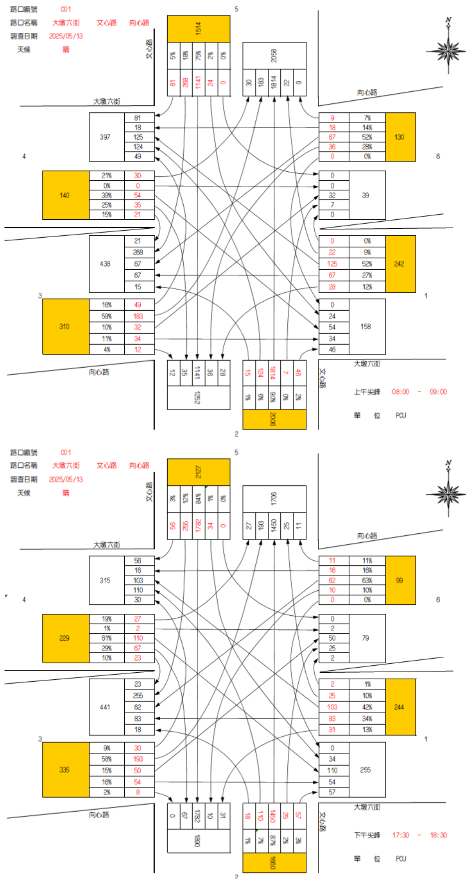
圖 1.1-2 大墩六街/文心路/向心路平日晨昏峰路口轉向交通量示意圖
