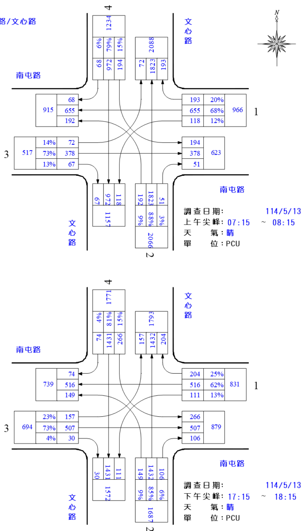
圖 1.1-4 南屯路/文心路平日晨昏峰路口轉向交通量示意圖
