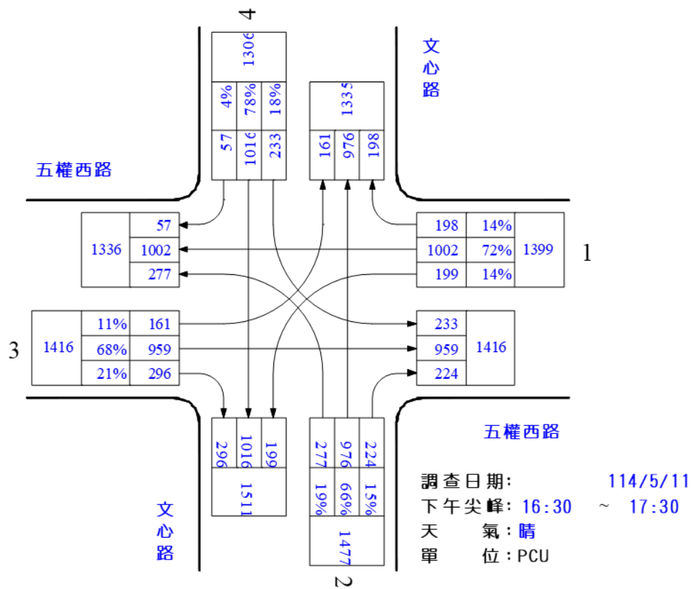
圖 1.1-8 五權西路/文心路假日晨昏峰路口轉向交通量示意圖
