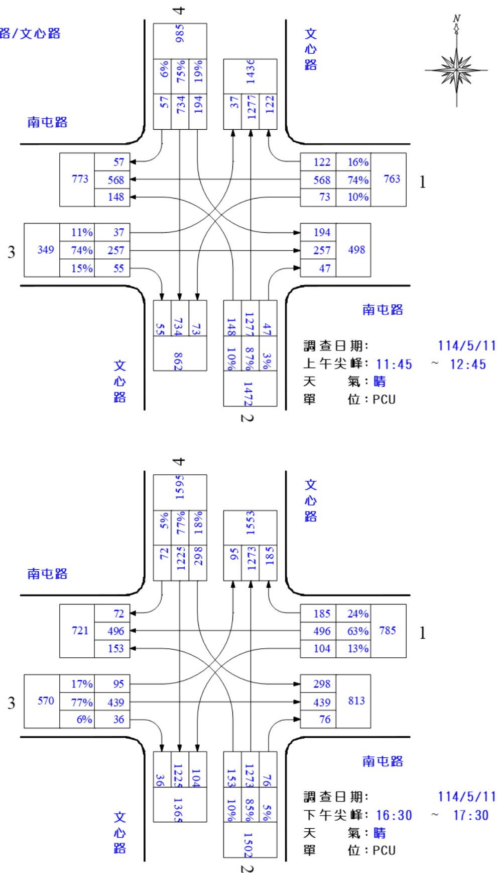
圖 1.1-9 南屯路/文心路假日晨昏峰路口轉向交通量示意圖
