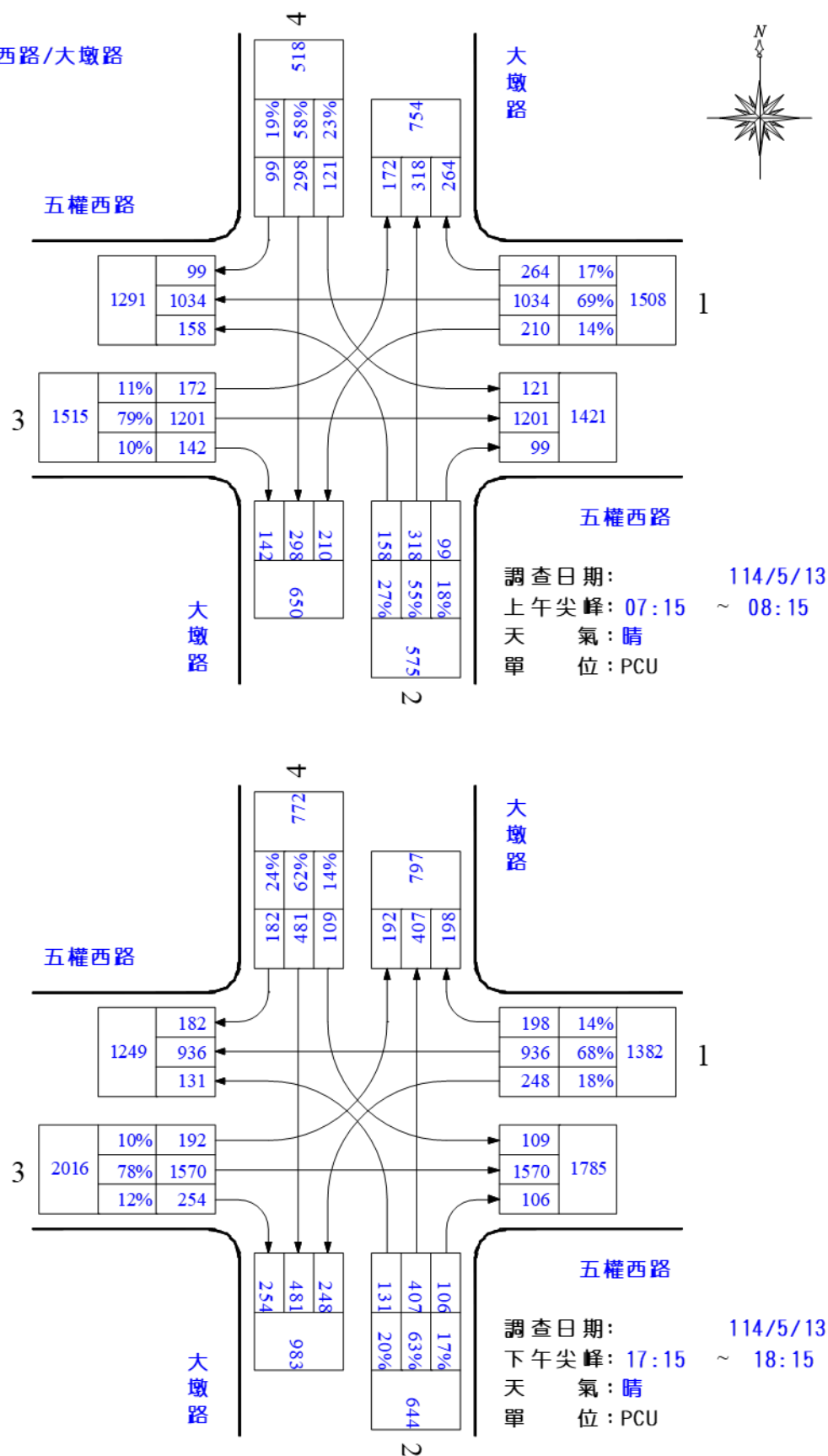
圖 1.1-6 五權西路/大墩路平日晨昏峰路口轉向交通量示意圖
