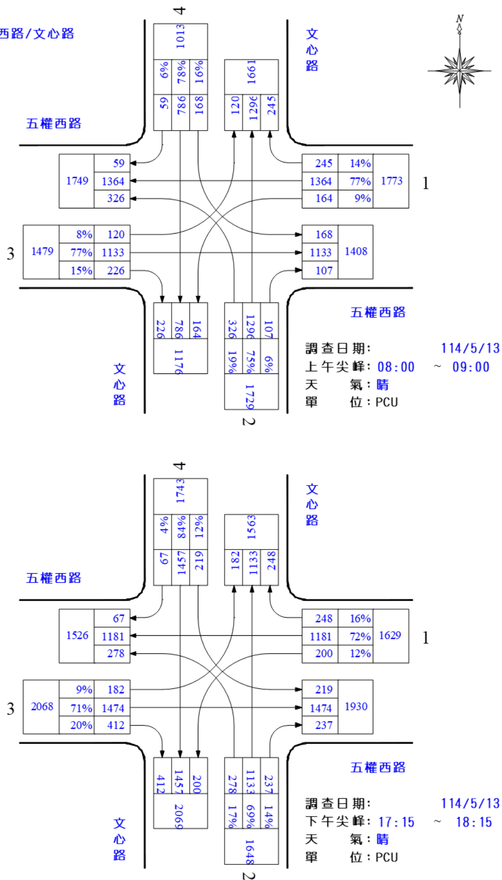
圖 1.1-3 五權西路/文心路平日晨昏峰路口轉向交通量示意圖
